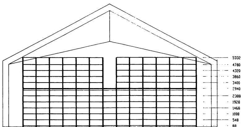
Tværsnit af det store reolssystem i det nyindrettede eksercerhus (Landsarkivet for Nordjylland).
