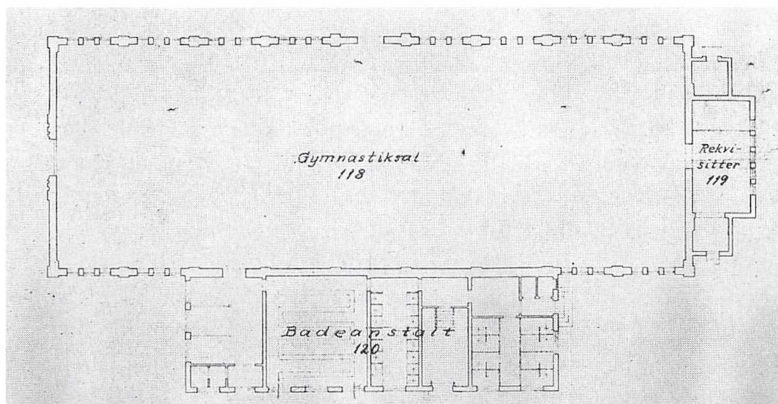
Plan over den tilbyggede badeanstalt (Forsvarets Bygningstjeneste, Viborg).
