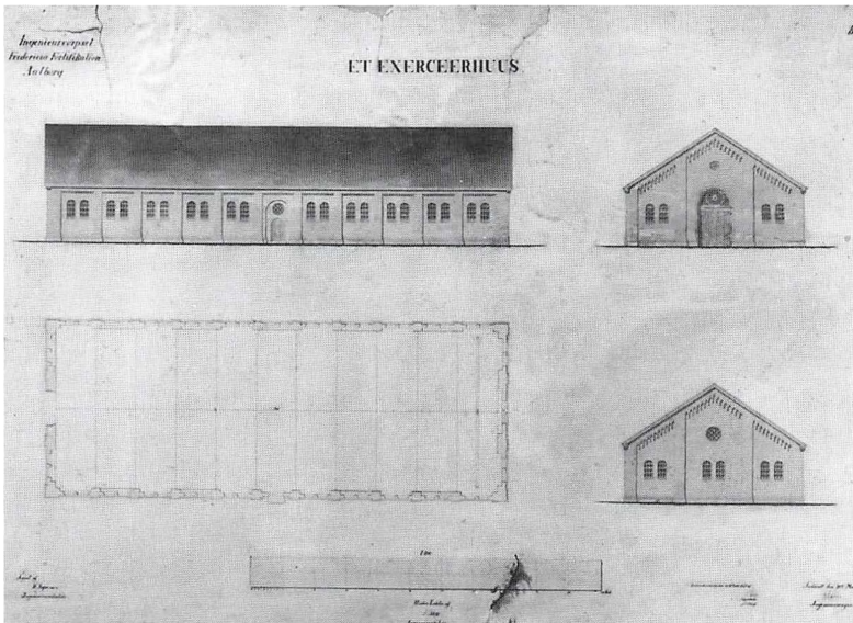
Plantegningen, som har titlen ET EKSERCERHUS, er udført af Ingeniørkorpset i 1866, og det er identisk med det i 1863 opførte hus i Fredericia. Med udsigten til opførelse af flere huse må huset i Fredericia være blevet gjort til forbillede. Uret over døren i gavlen blev taget som krigsbytte af østrigerne i 1864, og hullet har siden været lukket af en grøn plade. (Forsvarets Bygningstjeneste, Viborg).
