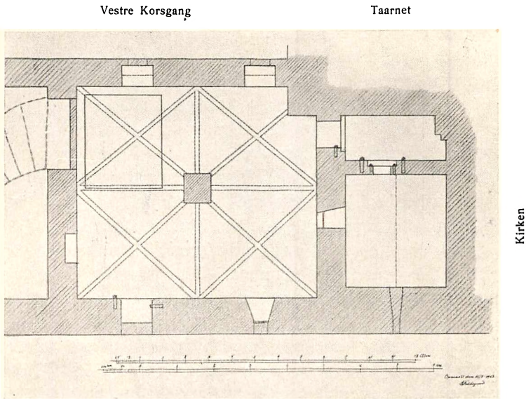
Afb. 3. Grundplan af Kælderpartiet (Vestsiden nedad).
