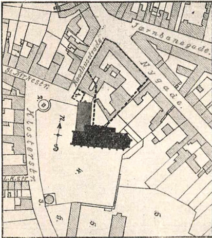
Afb. 2. Situationsplan.
