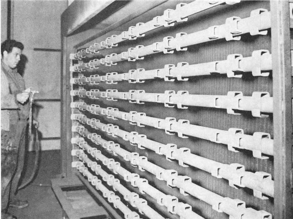
Elektrostatisk maling.
