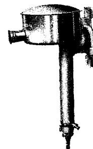
Destillationsapparat Model „DESTIL“ elektrisk Kapacitet: 6000 slag i timen
