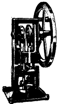
Håndtabletmaskine Model „HANTAB“ Max. tabletdiameter 12 mm Kapacitet: 6000 slag i timen
