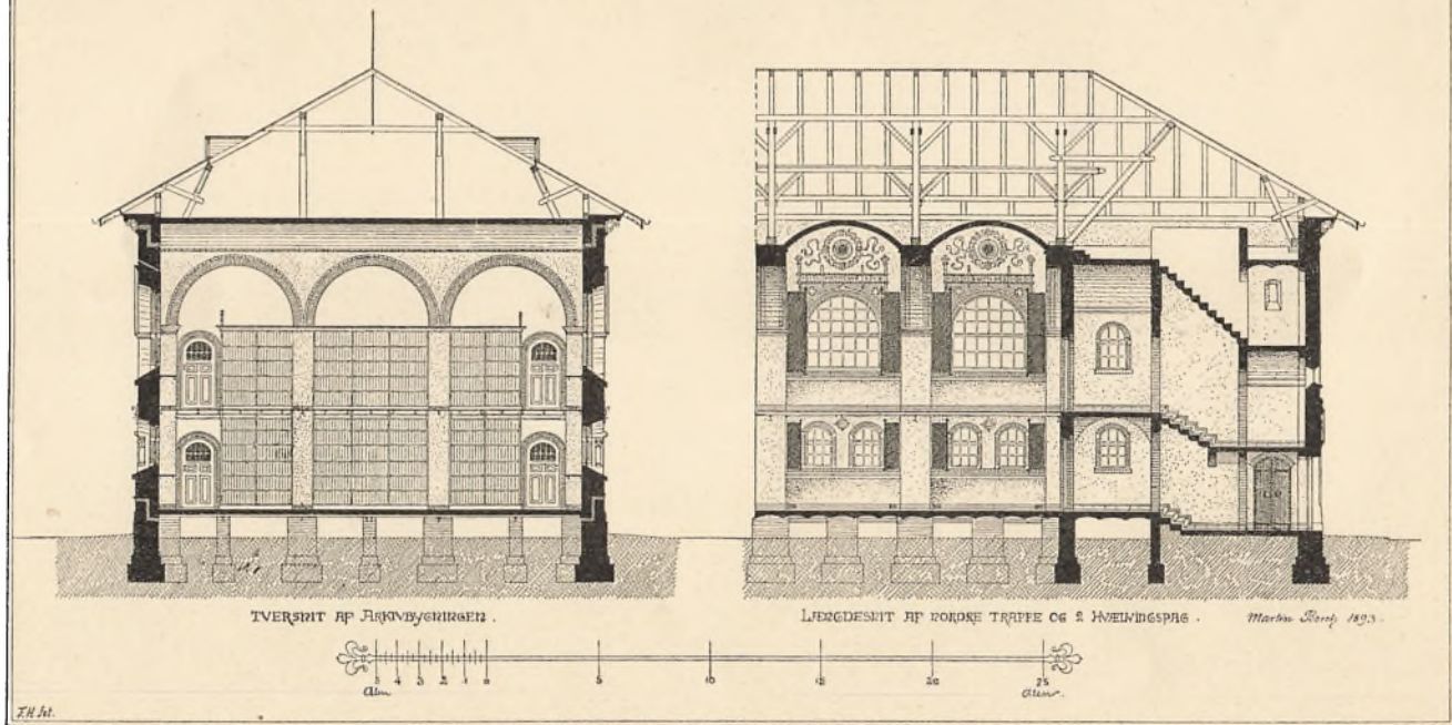
Tværsnit og delvist Længdesnit af Arkivet i Odense.
