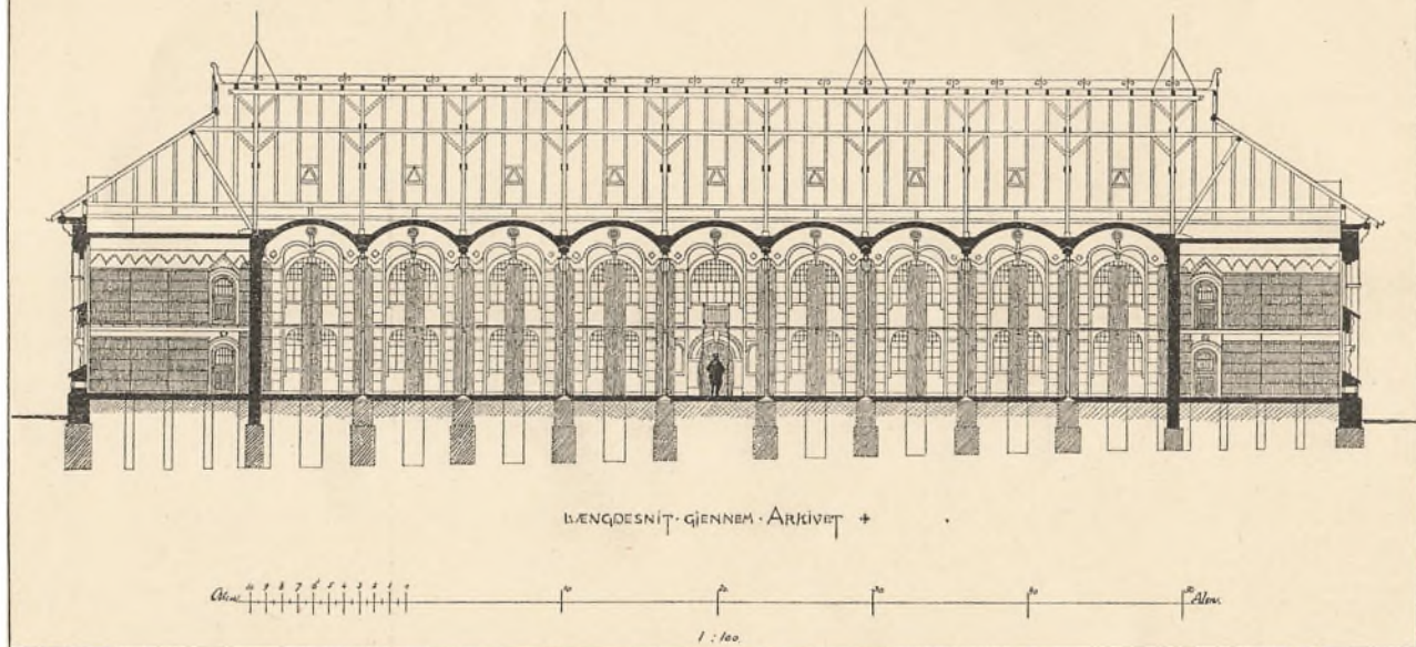
Længdesnit gennem Arkivet i Viborg.
