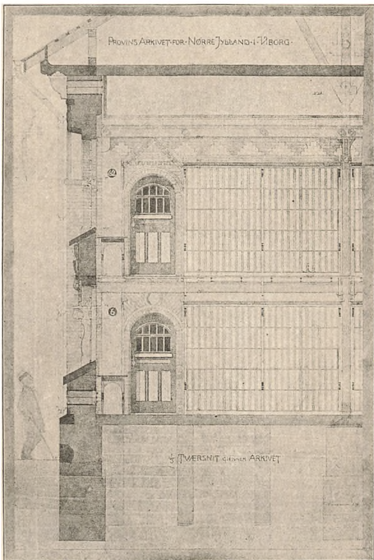
En Trediedel Tværnit gennem Arkivet i Viborg.
