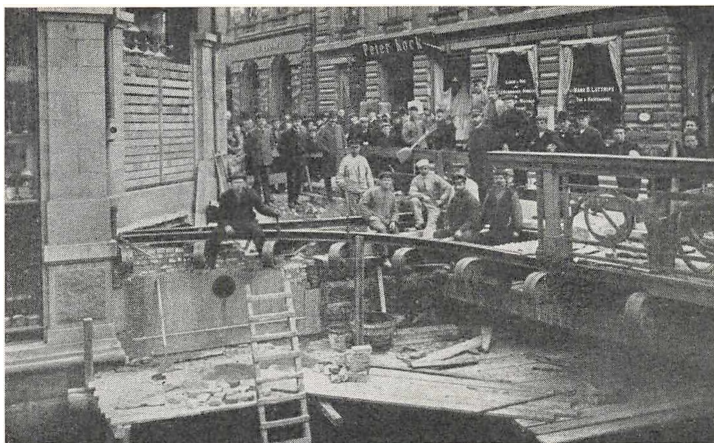
Skt. Clemens Bro set mod Søndergade. Anbringelse af stikbro ved Ankerhus. Stående nr. 3 fra v. stadsingeniør Oscar Jørgensen. Omkr. 1905
