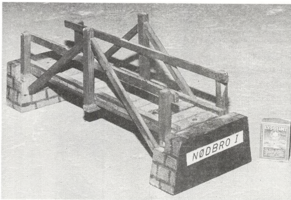
Undervisningsmodel af en mindre nødbro "Improviseret Bro"
