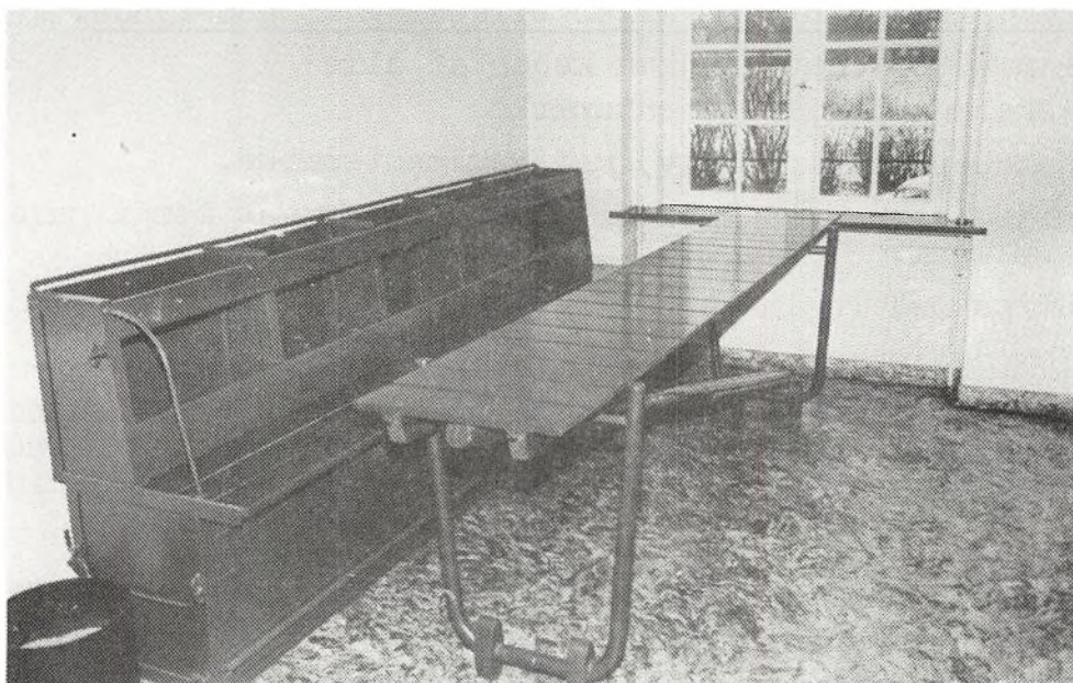
Venteplads foran regimentskontorer. Gammelt ingeniørmateriel. Bæk fra gruppepakning. Bordpladen er et stormspangsfæg på et stativ af bæksebom og vippebomme til brug ved bygning af en DIP - bro.
