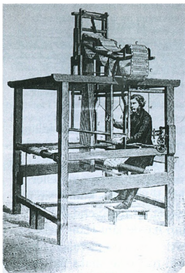
Jacquard-væven var forløberen for al industriel vævning, idet den styrede hulkortmønstreet automatisk. Den var konstrueret af den franske væver, Joseph Maria Jacquard (1752-1834). Industrialiseringen af væveteknikken nåede Danmark i 1830'erne og sendte håndvævere i massevis på landevejen. (Foto fra Sydsjællands Museum 1996).
