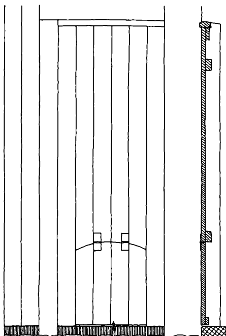
Gåselem. 1:20, Blegerstræde 2. (Opm. PA).
