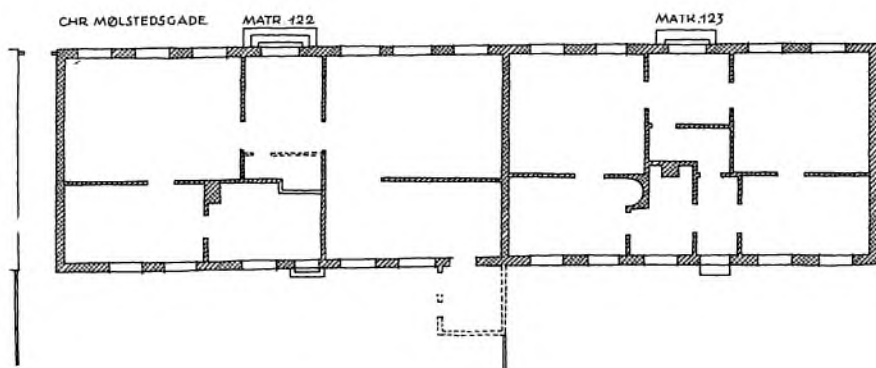
Chr. Mølstedsgade 5, matr. 122 og nr. 7, matr. 123. Begge huse opf. efter 1800-tallets midte. Den forøgede husdybde (omkr. 10\frac{3}{4} alen) og husenes to frie facader tillader langsgående skillevægge. Forbindelsen forstue-køkken er brudt ved senere tilføjede trapper. Plan og facader ca. 1:250. (Opn. P. E. N. Hansen, 1946).
