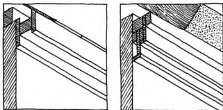
»Murede« gesimser udført af brædder. Chr. Mølstedsgade 3 og Vestgrønningen 34. (Opm. PA).
