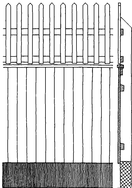
Plankeværk med stakit, 1:20, Kongevejen 12. (Opm. forf.).
