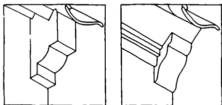
Gavlafslutning med udkrægning, 1:20. T.v. Kongevejen 9, t.h. Bymandsgade 30 (nordre tilbygning). (Opm. PA).
