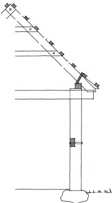
Bindingsværksdetaljer i Dragør: udvendig opstalt og snit. Opm. af Kunstakademiet 1946.
