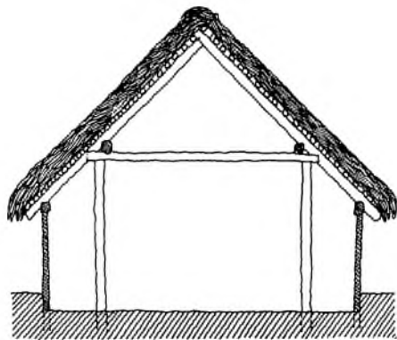
Principskitse af grubehus.
