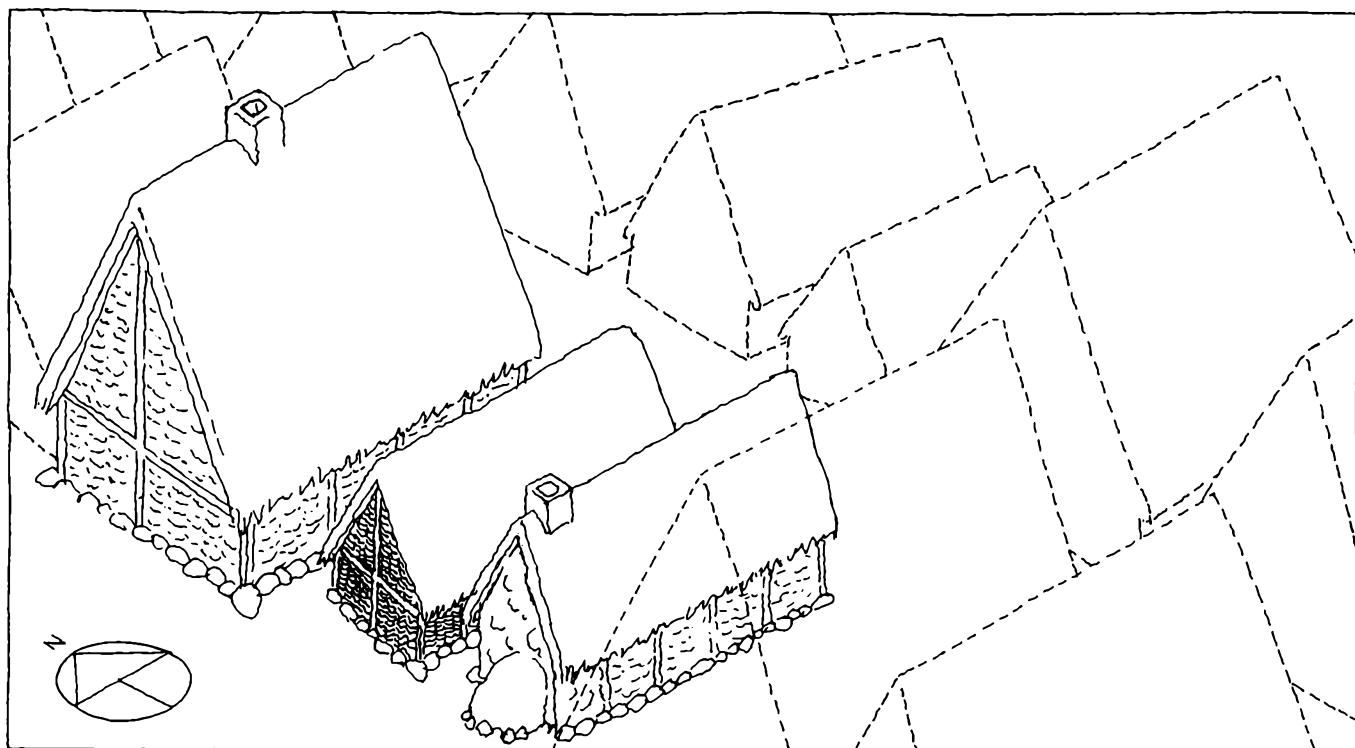
De tre gavlhuse i Nyenstræde, rekonstruktionsforsøg. (PA).
