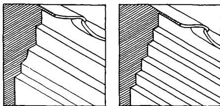
Blichmann-gesims, 1:20. Øverst l.v. Zylfensgade 4, t.h. Badstuevælen 8, nederst l.v. Vestgrønningen 3, t.h. Magstræde 3-5. (Opm. PA).
