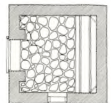
Beghuset, Dragør havneplads; benyttedes til kogning af beg i forbindelse med kalfatring; anvendtes tillige som køkken for ikke-hjemmehørende skibe, idet åben ild ombord var forbudt, når skibet lå i havn. Opstalt og snit, 1:100. Ildbænken er rekonstrueret. (Opm. PA)
