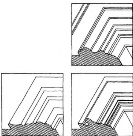
Dørindfatninger. Øverst Strandstræde 33, ca. 1750; nederst Vestgrønningen 18, ca. 1790; 1:5. (Opm. PA).
