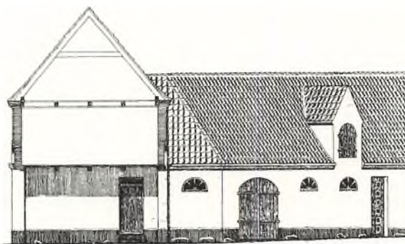
Snit i portbygning.
