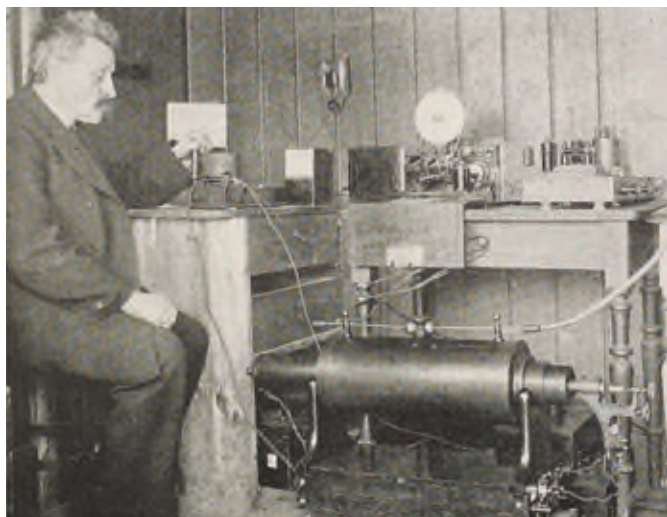
Fig. 5. Telegrafering uden tråd. Ferd. E. Sørensen eksperimenterer fra stationen på Kronborg 1901. (Illustreret Tidende nr. 3, 20. oktober 1901, s. 46)
