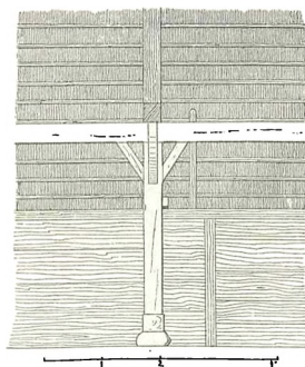
Fig. 250—252. Enkeltheder af Bulhuset i Emmerlev. (Se S. 213). Hovedskibet har intet Fodstykke. Stolperne støttes af Skraastivere og holdes sammen af Remmen. Der er kun en Bjælke i hvert andet Fag og ikke flere end fire fritliggende, skønt Laden er over 40 Alen lang. (Se Fig. 249). Sidevæggene, der er meget svage, holdes kun oppe ved spinkle Stænger, som gaar fra Remstykkerne til Hovedstolperne. Paa Fig. 252 ses en Hovedstolpe forfra og bag denne Dele af Væg og Tag.
