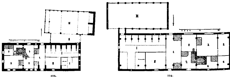
Fig. 111. Amrom. Fra det 18de Aarhundrede, Fig. 112. Før. Fra det 17de Aarhundrede. Den skraverede Del af Ydervæggen er af Rør, Fig. 113 og 114. Fra Kornkøgen (Egnen mellem Husum og Tønder). Opførte kort efter Stormfloden 1634. (Jævnf. Fig. 102 og 104). I Stalde, II Loer, III Lade, IV Faaresti, V Svinesti, VI Bod, 1 Dile, 2 Stuer, 3 Pisel (Storstue), 4 Køkken, 5 Kamre, 6 Kældere. Øvret bæres af jordgravede Stolper, der staar 1 til 2 Alen indenfor Ydervæggene og i Planerne er angivne ved smaa sorte Kvadrater. I Fig. 113 og 115 er disse Stolper ved Murværk forbundne med Ydervæggene. Jævnf. Fig. 78 til 82.
