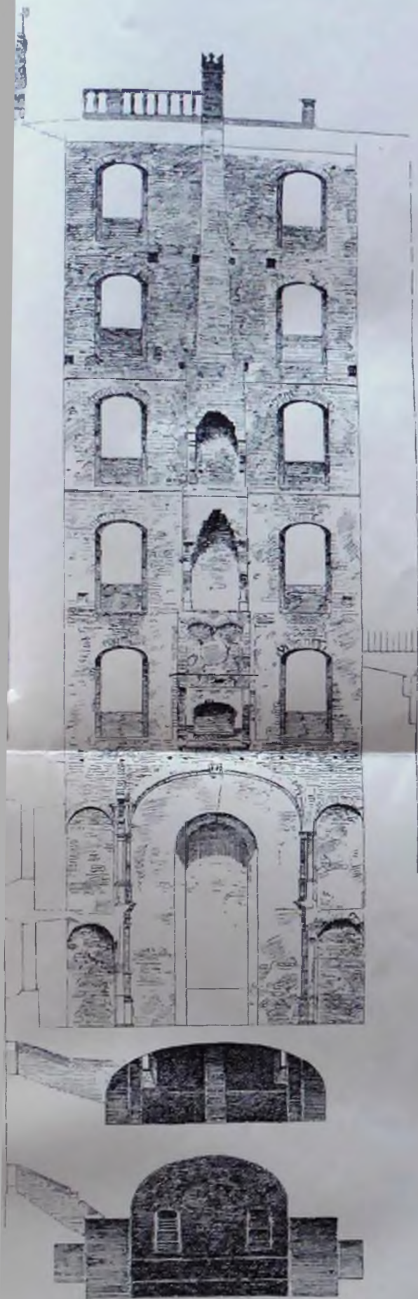
Snit af Kæmpetaarnet, (Vest-Øst).
