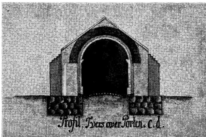
Profil af Prinsens Port, tegnet 1754 af S. C. Gedde (note 22).
