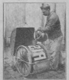
Ku ny Maade at reklamere paa. Den lille Vogn trykker Reklamer paa Gadenes Stenbro, men det er ikke med Farver, kun med Vand. For hver Vandpaafyldning kan Vognen trykke en 3 Kilometer lang Reklame. Men den kan altsaa kun anvendes, naar Gaden er fuldstændig tør. Man ser af de to Billeder til venstre til højre Reklamevogns Mekanik og til højre Vognen i Virksomhed paa en Gade i Paris.
