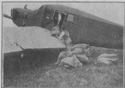
Den danske Amerikaner John Larsen, som vi flere Gange har set herhjemme med hans Flyvemaskine, har konstrueret en ny Maskine, der er helt af Metal. Der er ikke en Pind Træ i den. John Larsen har til den amerikanske Postforvaltning bygget en hel Serie af disse Maskiner, der skal besøge Postflyvningen mellem forskellige Byer i Staterne. Det er en af Maskinerne, man ser her.
