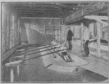
Og her er vi ved Øresund. Studenternes Roklub i København har i Kalkbrænderihavnen indrettet et Træningsbassin for Iboerne. Det er mauret i Cement, og man har det Fjeldl fra for Træning paa Søen, at Træningen her kan staa ved Siden af og rette Pælene. Sæderne kan drøjes, saa man baade kan ro styrbords og bagbord, og Aarslagene driver Vandet rundt i en Omlobskanal, saa den nødvendige Modstand opstaar.
