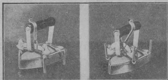
Dette elektriske Strygejern kan ikke tænde Ild, selv om man sætter det fra sig og har glemt at skruer Kontakten om. Det er nemlig forsynet med en lille Anordning, hvorefter man kan give det fire Fodder at staa paa, naar det er ude af Brug. Til venstre ses Fodderne slæede med, til højre Jærnet i Arbejde. Opfundet af Joh. Bjørnshof, Alexandrævej 16, København.
