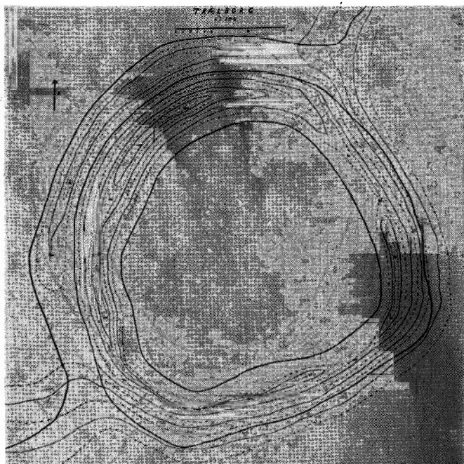
Fladenivellement og Opmaaling af Trælborg Voldsted 1954.
