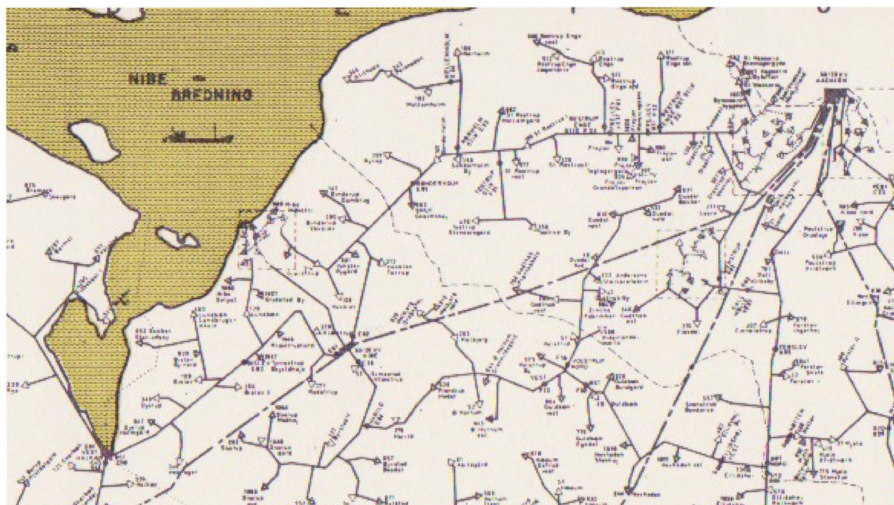
Figur 105: El-nettet i Vokslev Sogn, 1972. Transformationer angivet med trekant.
