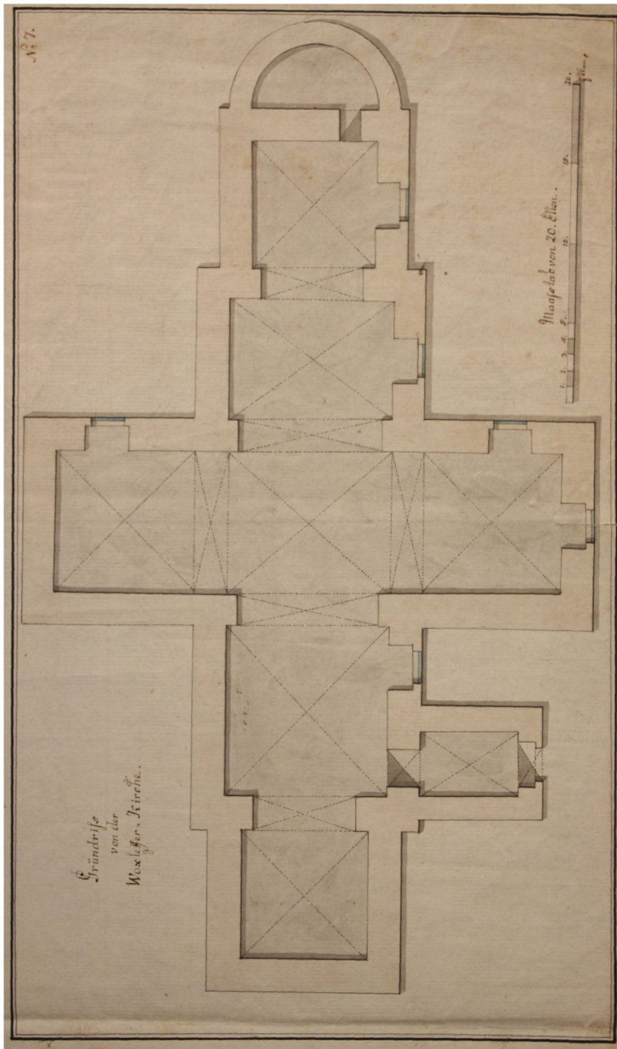
Figur 64: Vokslev Kirke, plan formodentlig fra 1768. Teksterne er på tysk. Korsarmen mod syd nedbrudt 1815. Aalborg Vestre Provsti, Nibe.
