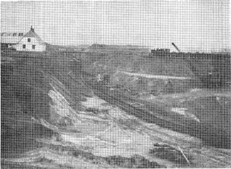
Lejet ved FASTERLUND. Ved gården ses vejbroen med Astrup-Ejstrup landevejen. Herunder føres tipvognssporet fra graven op til læsserampen ved DSB-sporet. Tipvognskolonnen i baggrunden flytter overjord.
