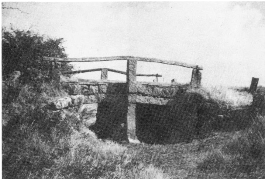
Immervad bro sydvest for Haderslev, opført 1786, og af samme type som Smedevadbro. Broen ved Immervad er bevaret uændret, men har mistet sit vandløb.
