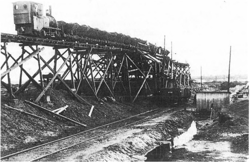
Høj læsserampe ved Nørre Vium brunkulsleje i 1943. (S. A. Guldvang: Danmarks smalsporede industribaner. 1988).
