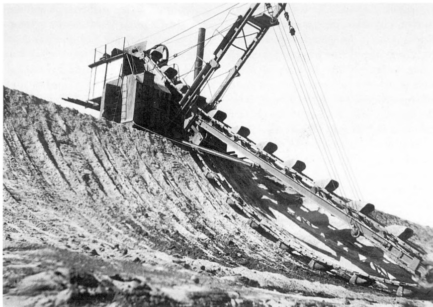
Nr. Vium-lejet. Spandkædegravemaskine.
