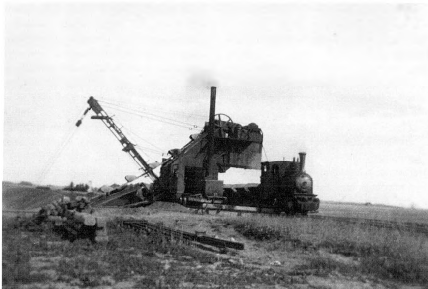
Ejstrup-lejet. Dampdrevet spandekedegraver fylder en kolonne tipvogne med overjord. 1943. (Foto: Henry Jørgensen).
