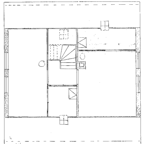
Plan af Sagstagen.
