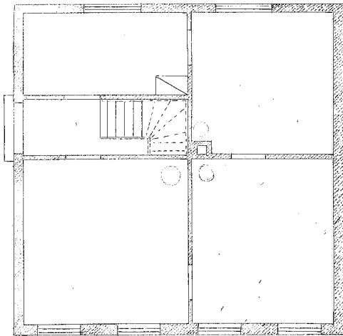
Plan af Stuen.
