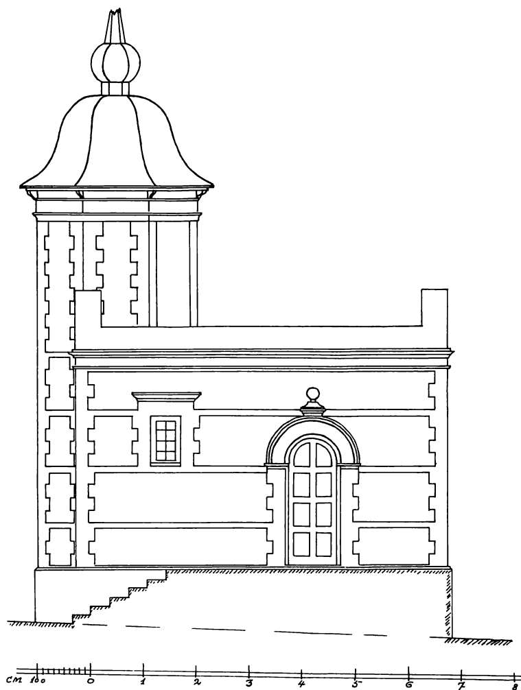
Øst. Planer, snit og façadeer, efter opmåling af arkitekt J. Tidemand-Dal, m. a. a. 1938.
