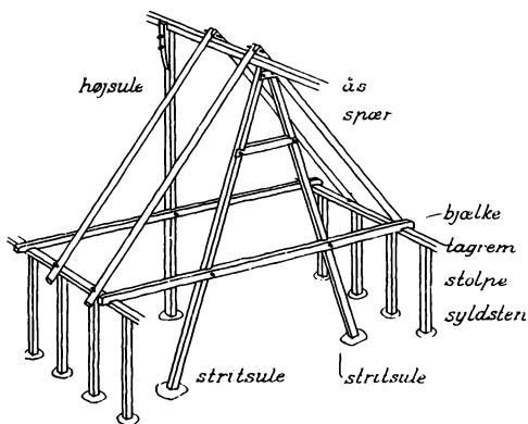
Konstruktion med højsule og stritsule. Suler° og stolper° står direkte på syldstenene°
