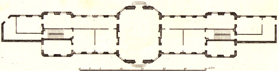
GRUNDPLAN AF NEDERSTE ETAGE.
