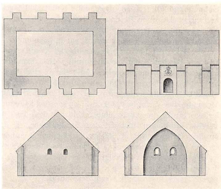
2. Grundrids, vestre Facade, Gavl og Tværsnit af Krudttaarnet i Grevens Bastion. Tegning i Ingeniørkorpsets hist. Kortsaml.
