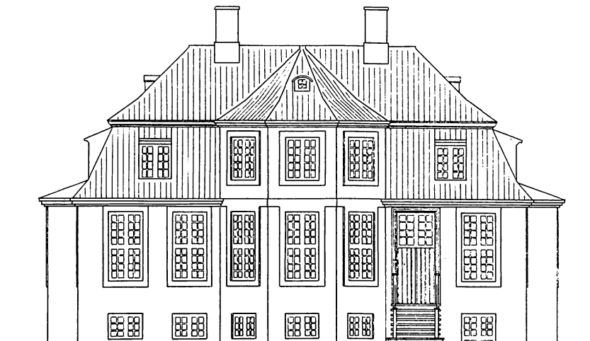
Fig. 2. Gaardfaçade. Opmaaling af Teknisk Skoles Bygningskole 1927—28. 1 : 200.
