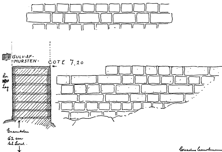
4. Rester af Muren om Auditoriebygningen. Tegning.
