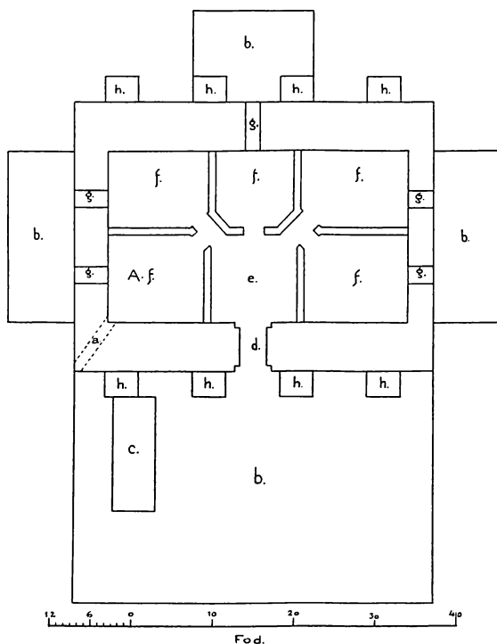
3. Grundrids af Krudttaarnet i Grevens Bastion. Tegning i Hærens Arkiv.
