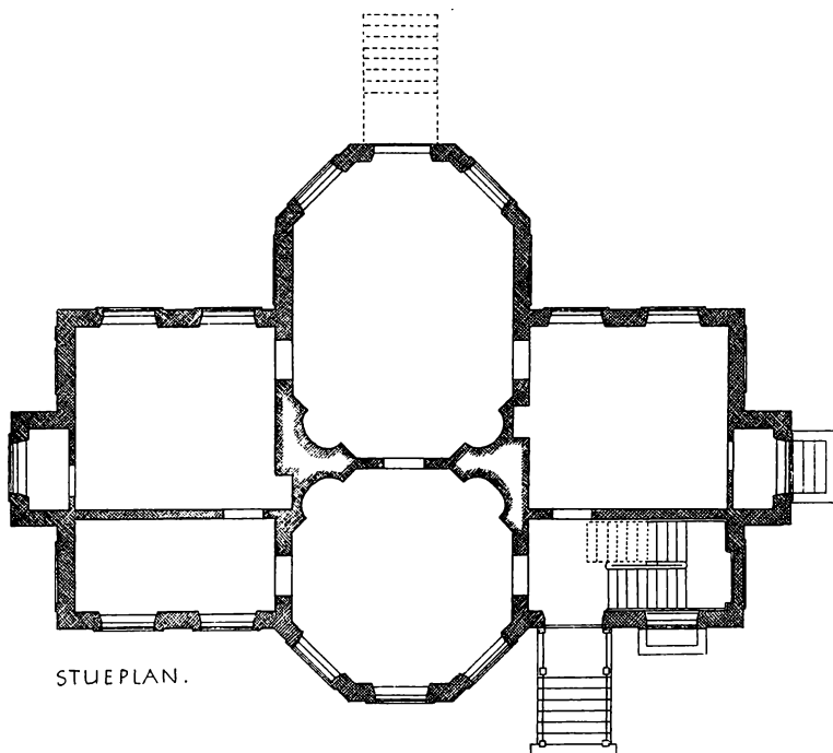
Fig. 3. Stueplan. Opmaaling af Teknisk Skoles Bygningsskole 1927—28. 1 : 200.
