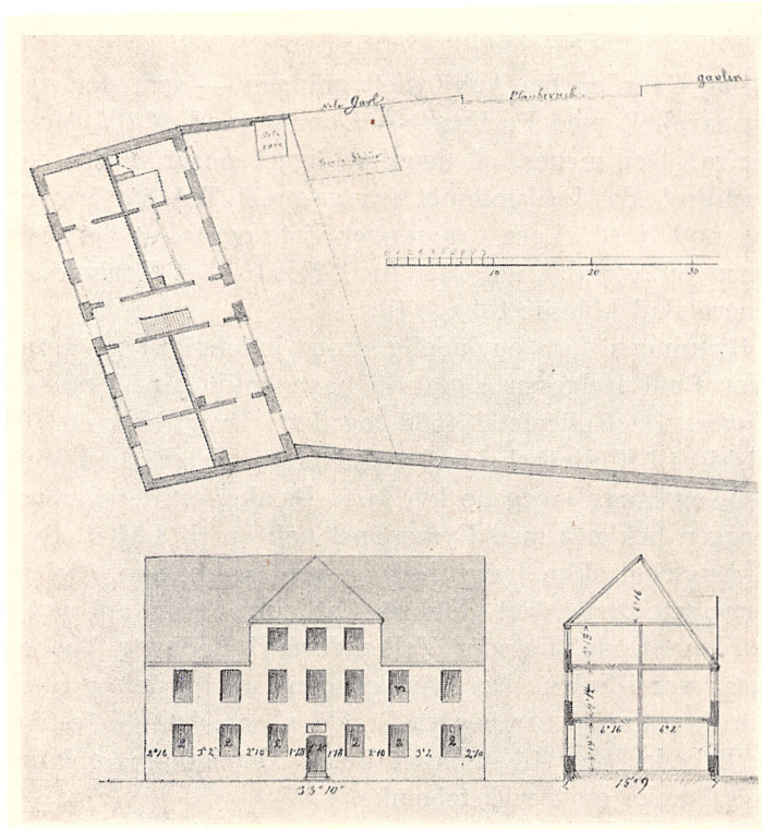
3. Opmaaling af Kollegiet før Nedrivningen i 1865. Kgl. Bibl. Kortsaml.
