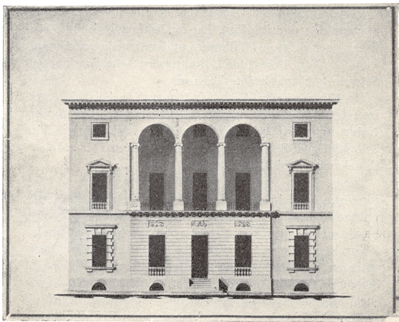
Palmille 49. Sydside. Originaltegning af C. F. Hansen. Kunstakademiet. Efter „Samleren“.
