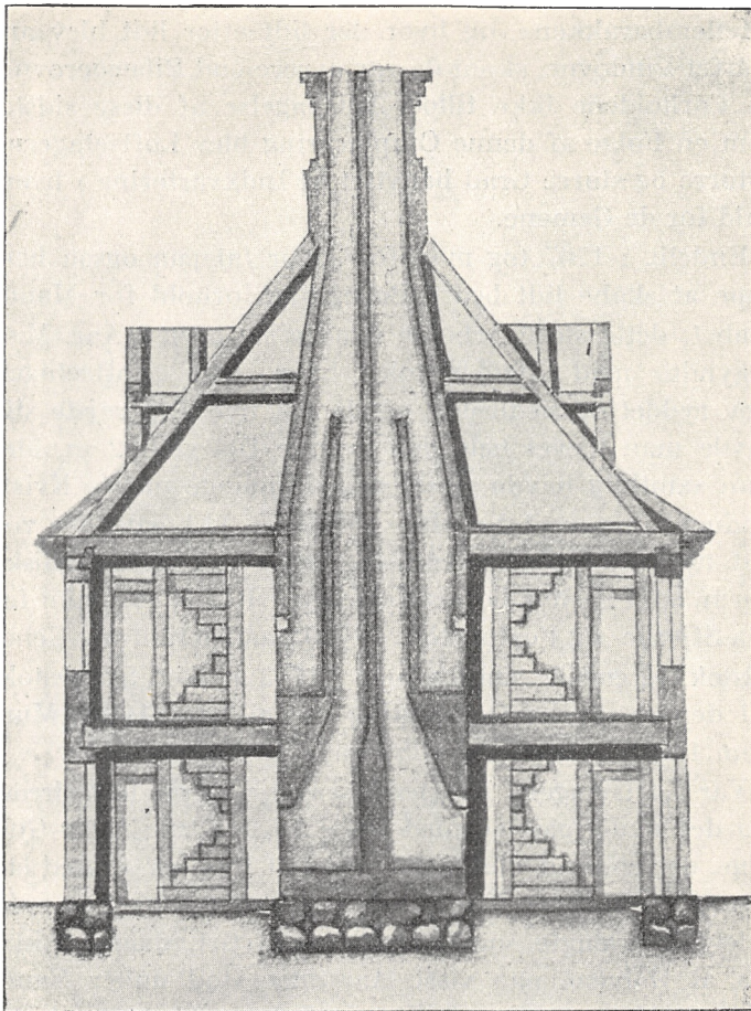
Tværsnit gennem en Dobbelbarakke. Se S. 211.
