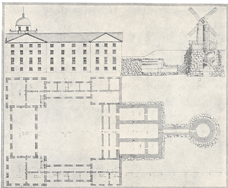
Nordre Sidefaçade og Grundrids af det projekterede Slot i Kastellet.
