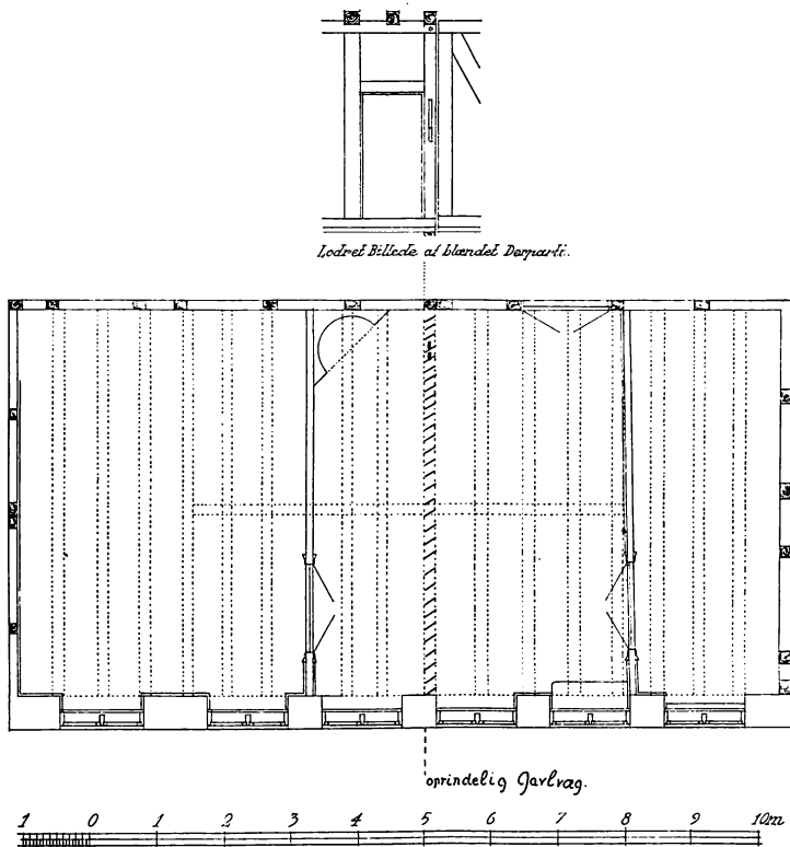
Brogade 3. Plan af 1. Sal.
