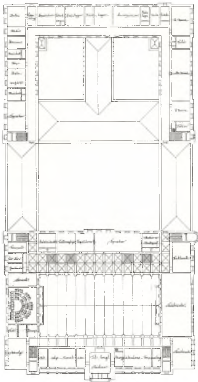
L. Fengers 2. projekt 1888, plan af 2. sal. Facaden nedad. 1:ca. 900.
