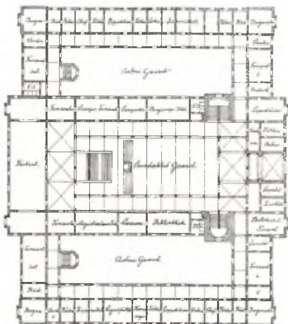
M. Nyrops skitse I A 1891, plan af 1. sal. Facaden mod højre. 1:ca. 1200.
