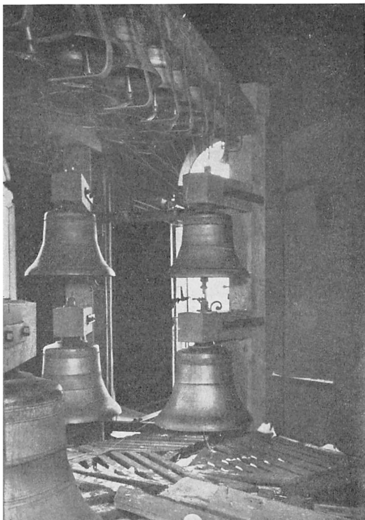
Klokkespil (Vor Frelzers Kirke, Kbh.) med tilhørende mekaniske Træk. Man ser tydeligt Metaltraadene, hvorved Kneblerne i de enkelte Klokker sættes i Bevægelse. Traadene fører til Klaviaturet, der findes i et Rum længere nede i Taarnet.
