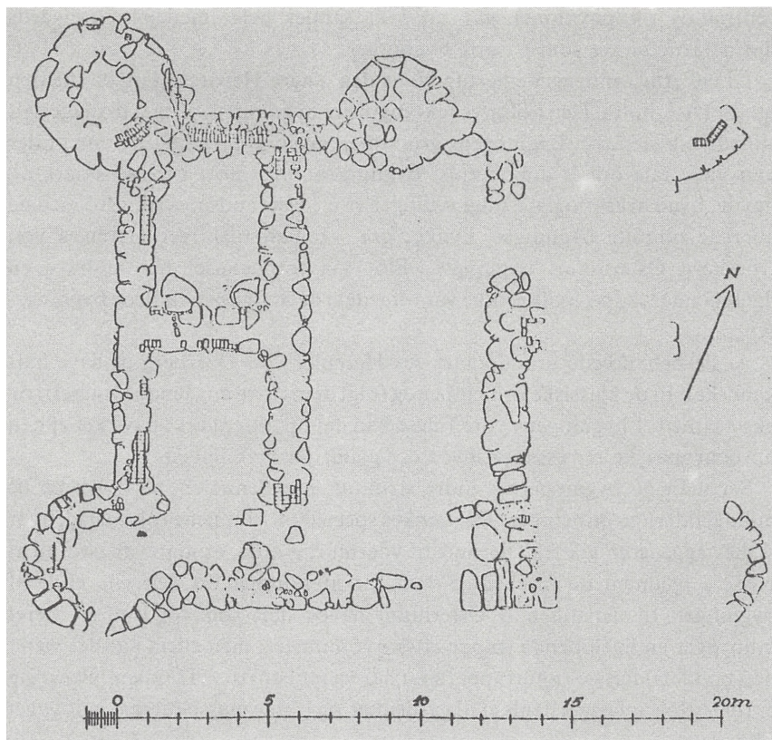
Fig. 5. Grøngårds grundplan. (Efter Nationalmuseets Arbejdsmark 1956).
