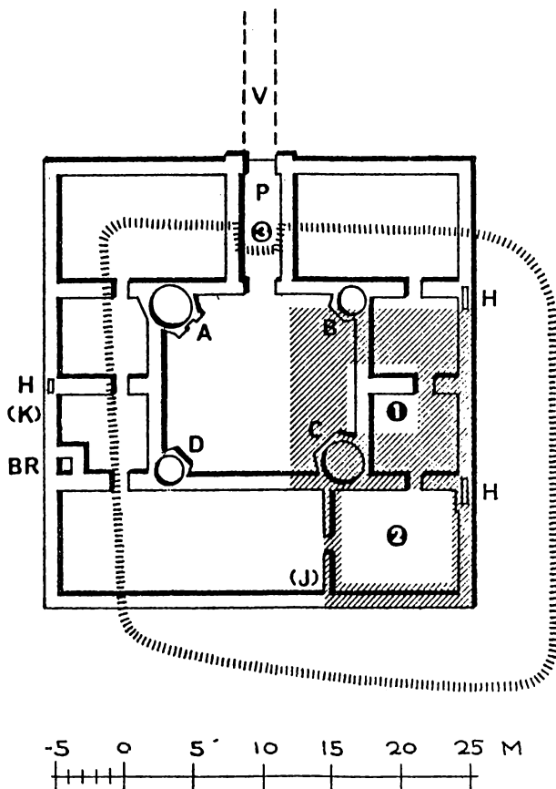
Fig. 2. Trøjborgs grundplan. (Efter Trap Danmark).
