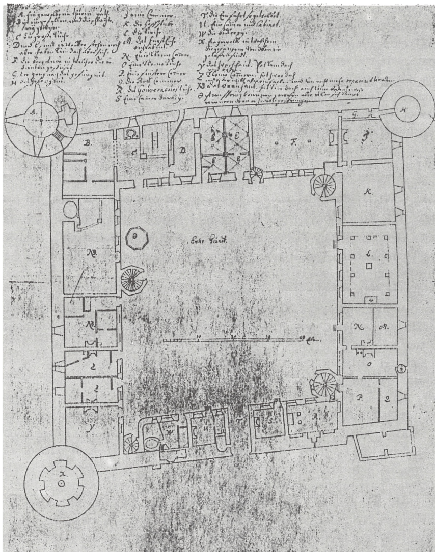
Fig. 4. Sønderborg Slot – planen af stueetagen. (Efter Otto Norn: Christian III's borge).
