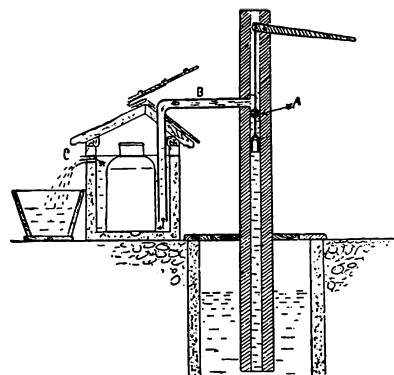
Skematisk fremstilling af mælke-kølebassin i forbindelse med vandpumpe og vandingsstrug.
