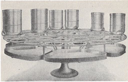
Buas resttømningsapparat. Efter at spandene var blevet tømt roterede de rundt med bunden i vejret. De dråber der endnu var til overs, blev opsamlet i et kar som vist på fotoet. Ellebrecht 1917 bd. IV. s. 431.
