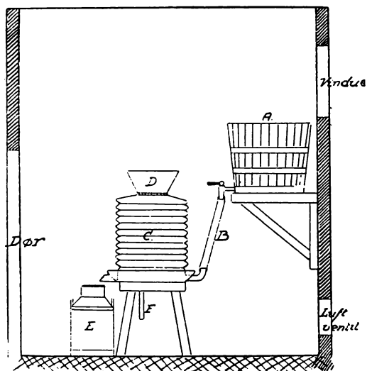
Skematisk fremstilling af mælkekøleanlæg med ringhøler. Vandet tilføres apparatet fra beholderen A og går op gennem apparatet, mælken hældes i tragten D og risler ned over ringene på køleapparatet. (Modstrømsprincippet).
