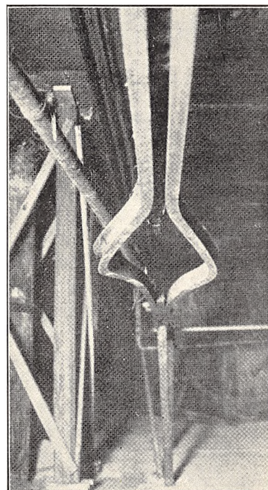
Fig. 2. Ubeskyttede Jernbjælker ud-bøjede efter Brand.
