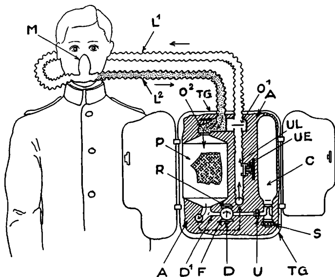
Fig. 48. Skematisk Fremstilling af Kredsløbet i Dräger K. G. 1928
