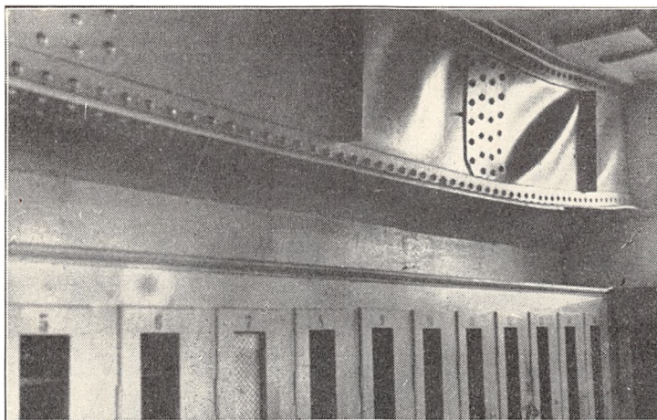
Fig. 1. Ubeskyttet Jerndrager, der har været udsat for Opvarmning fra en lokal Brand i Rummet.
