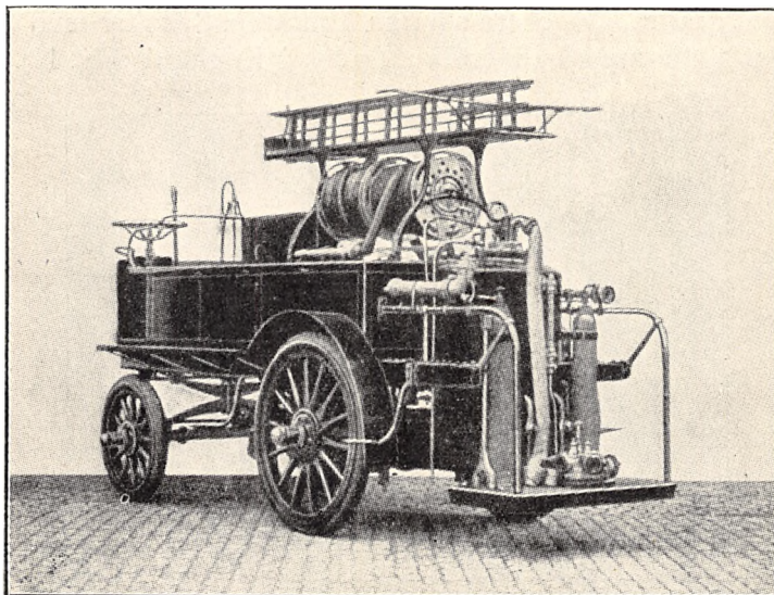
Fig. 13. Kulsyresprøjte.
