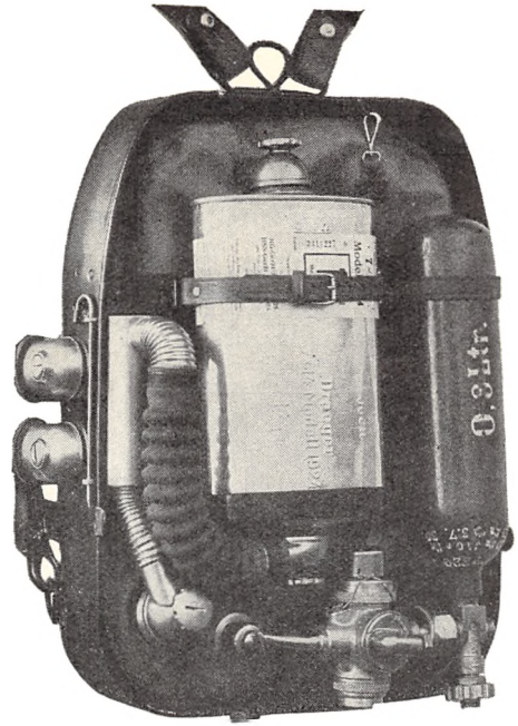
Fig. 50. Kredsløbapparat Model Dräger K. G. 1931
