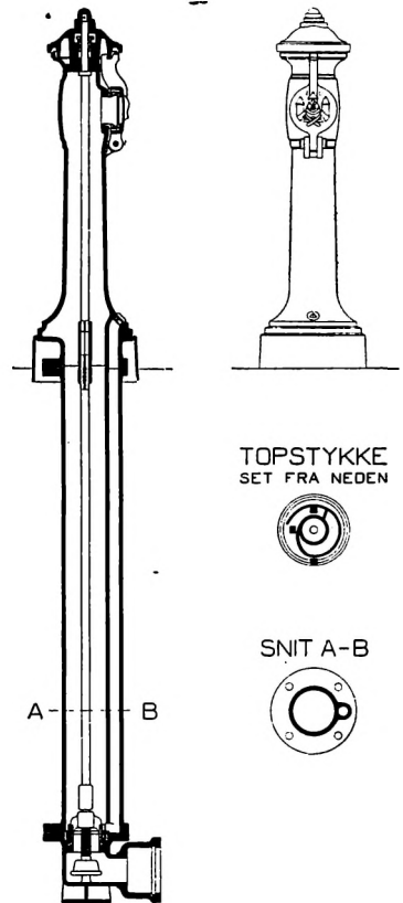
Fig. 52. K. V. Brandhanen.
