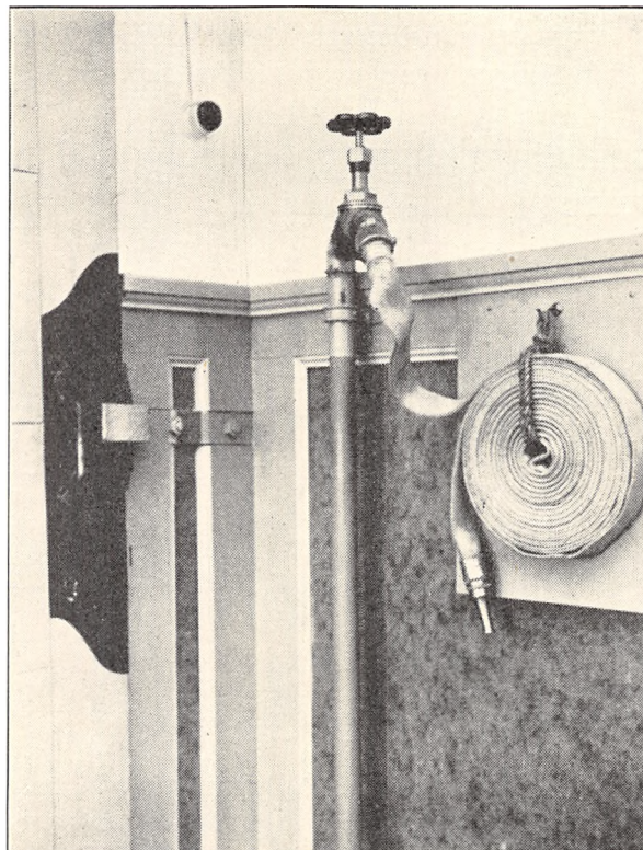
Fig. 14. Fra Midten oprullet Slange ophængt i Strop.
