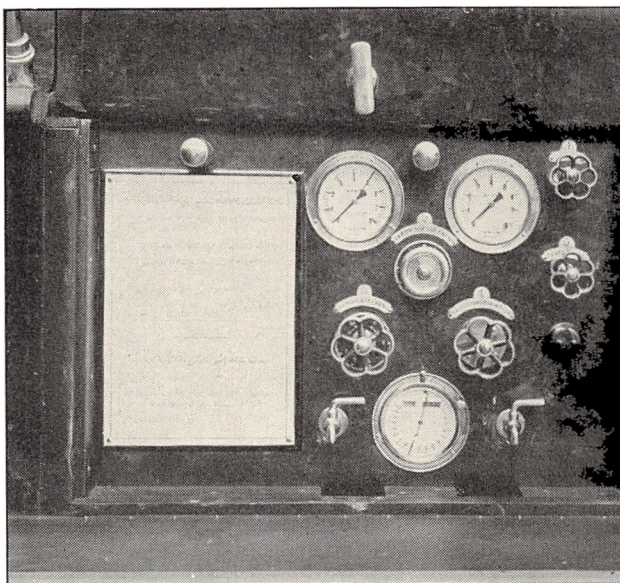
Fig. 24 a og b. Schröder og van Deurs Skumaggregat til en Motorsprøjte eller Motortender.
