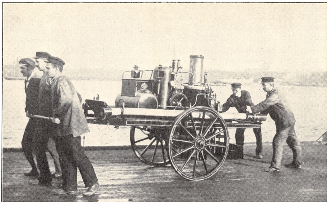
Fig. 7. Dampsprøjtetype fra Ludwigsbergs Werkstads A. B. Stockholm.
