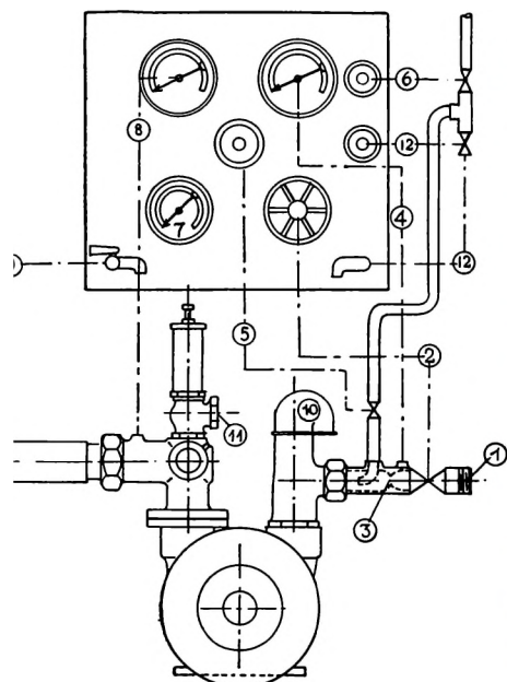
Fig. 24 a og b. Schröder og van Deurs Skumaggregat til en Motorsprøjte eller Motortender.
