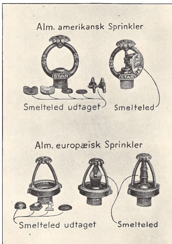
Fig. 16. Typer af Sprinklerhoveder.
