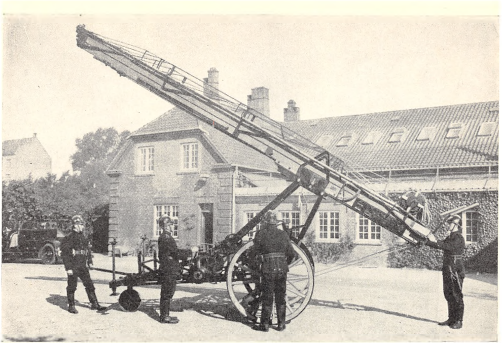
Fig. 35. En af Københavns Brandvæsens 22 m Afprotstiger Model 1930. Stigen afprotset.
