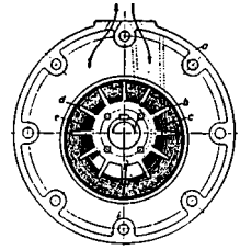
Fig. 17. Vandringsspumpe. a Pumpehus, b Løbehjul, c Sugeseide, d Vandring, e Trykside.
