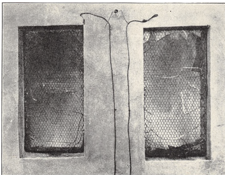
Fig. 10. Monierglasruder, der har været udsat for Brandpaavirkning i ca. \frac{1}{2} Time.
