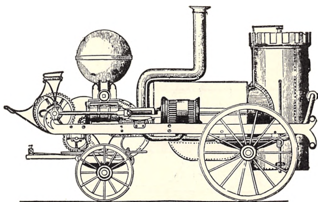
Fig. 4. Braithwaite og Ericssons Dampsprøjte 1829.
