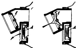
Fig. 45. Ventilene i S. Maskerne.
