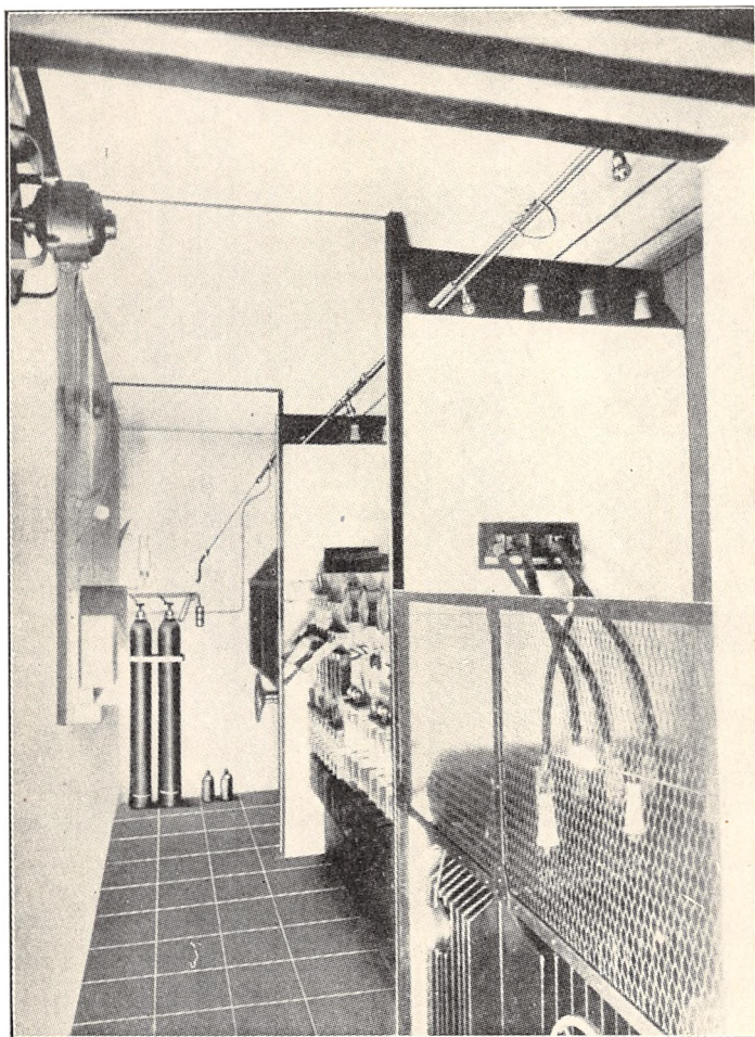
Fig. 26. Kulsyresanlæg i et Højspændingsrum.
