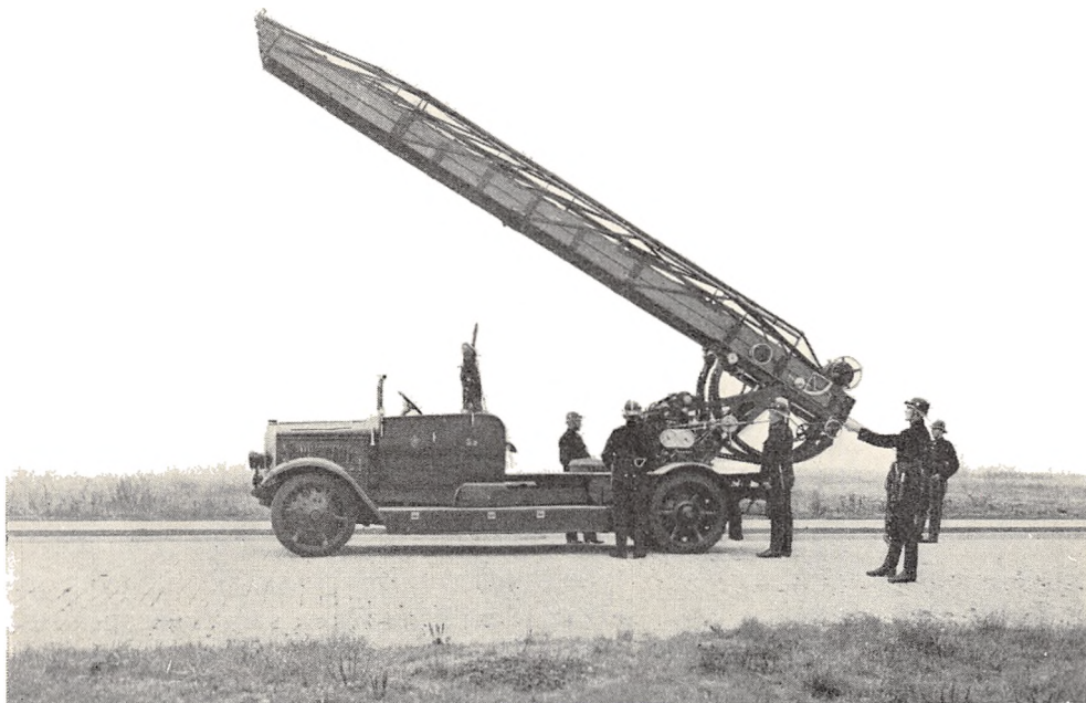
Fig. 33. Københavns Brandvæsens 28 m Taarnstige Model 1930.
