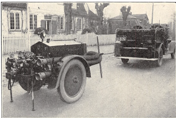
Fig. 21. Paahængsmotorsprøjte.
