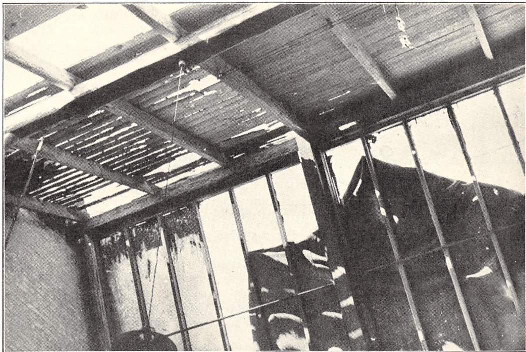
Fig. 7. De 3 Monierglasruder til venstre har holdt til en ret voldsom Brand.
