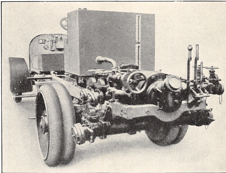
Fig. 16. Motorsprøjte med aftaget Karosseri.
