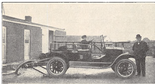
Fig. 22. Ellehammer Sprøjte.
