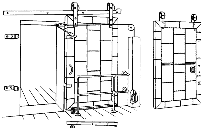
Fig. 11. Jernbeklædt Træ-Skydedør.
