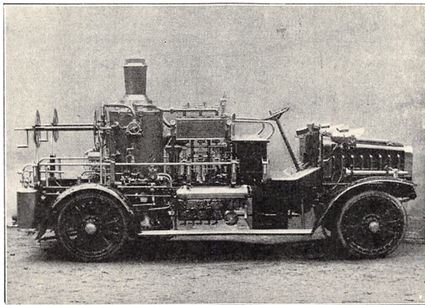
Fig. 9. Dampsprøjte monteret paa et Elektromobil Wien 1907.
