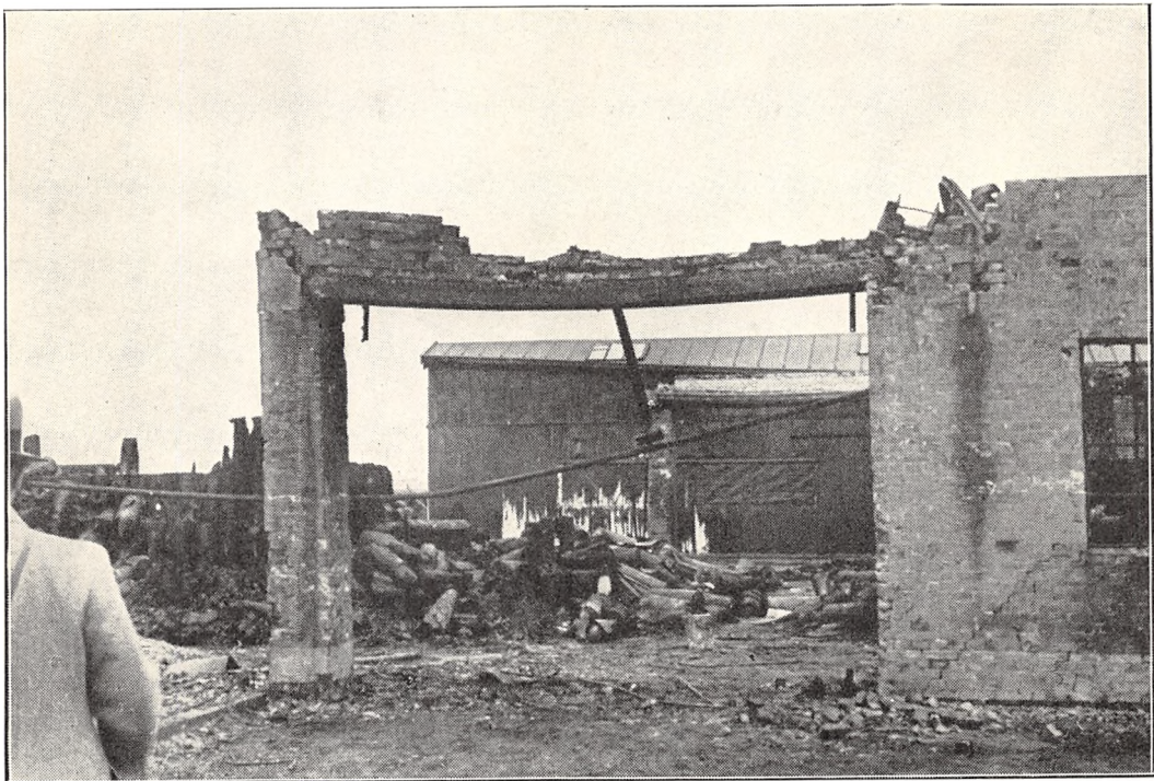
Fig. 3. Jernbjælke, der har sprængt Murværk ved Varmeudvidelse.
