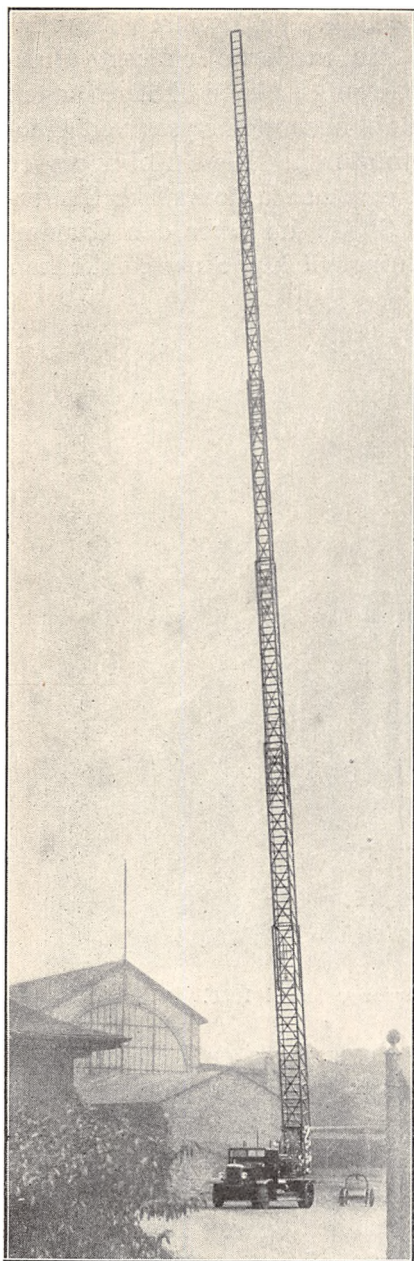
Fig. 34. 48 m Drejestige til Bruxelles Brandvæsen, leveret af Metz i Karlsruhe.
