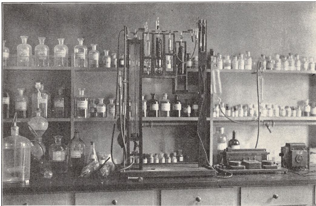
Fig. 55. Modificeret Orsat Apparat til Røganalyser.
