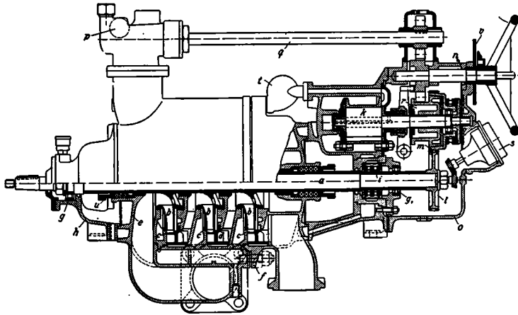
Fig. 15. Centrifugalpumpe til Motorsprøjte.
