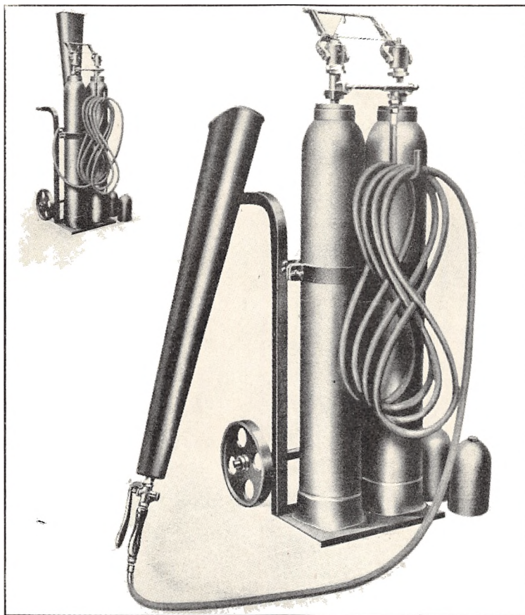
Fig. 25. Transportabelt Kulsyresneaggregat.
