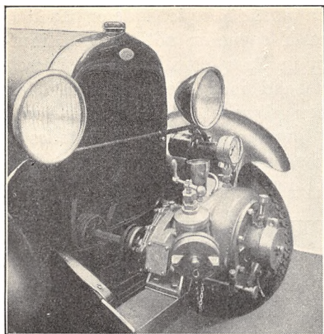
Fig. 20. Mindre Motorsprøjte med Pumpen foran Motoren.
