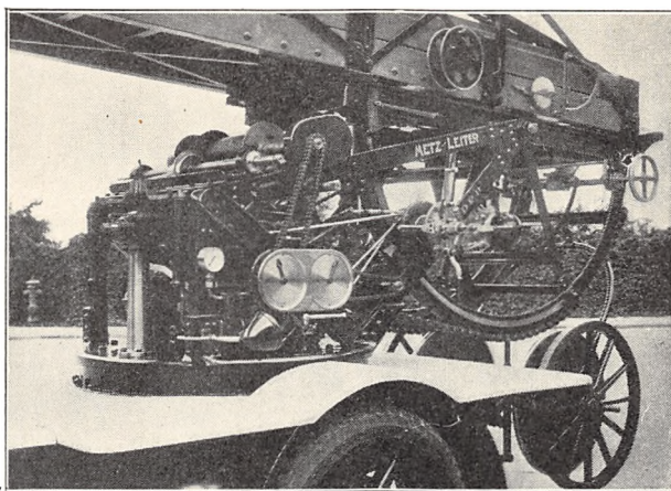
Fig. 31. Manøvreringsmekanismen paa Københavns Brandvæsens 28 m Taarnstige Model 1930.
