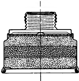
Fig. 42. Snit igennem et F. Filter. (Brandfilter).
