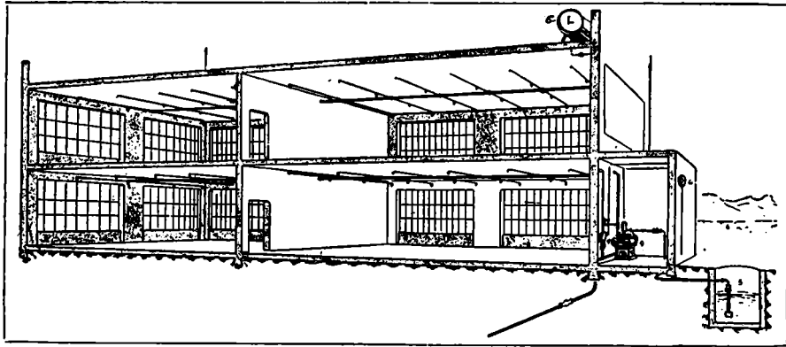
Fig. 17. Skematisk Sprinkleranlæg.
