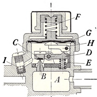
Fig. 47. Dräger Reduktionsventil.
