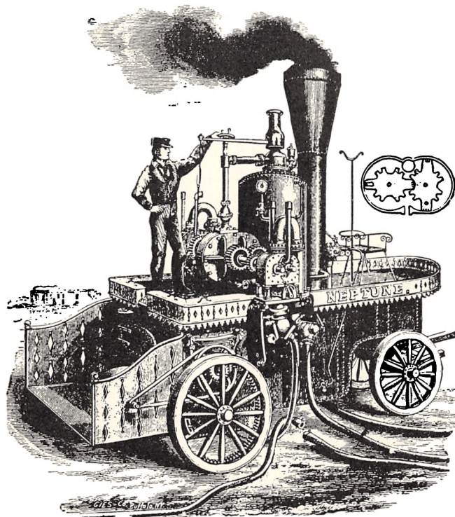
Fig. 6. The Silsby Manufacturing Companys Dampsprøjte 1856.
