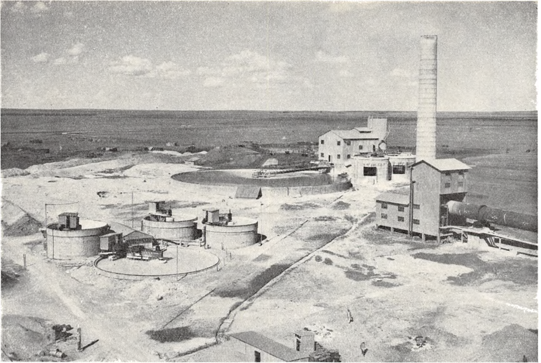
Cementfabrik i Sydafrika, bygget af F. L. Smidth & Co.
