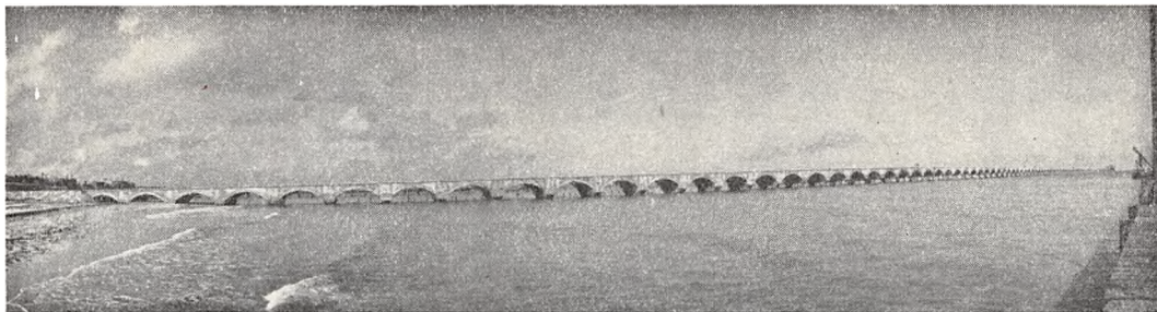
Den 2100 m lange Pier ved El Progreso, Yucatan, Mexico. Udført af Christiani & Nielsen
