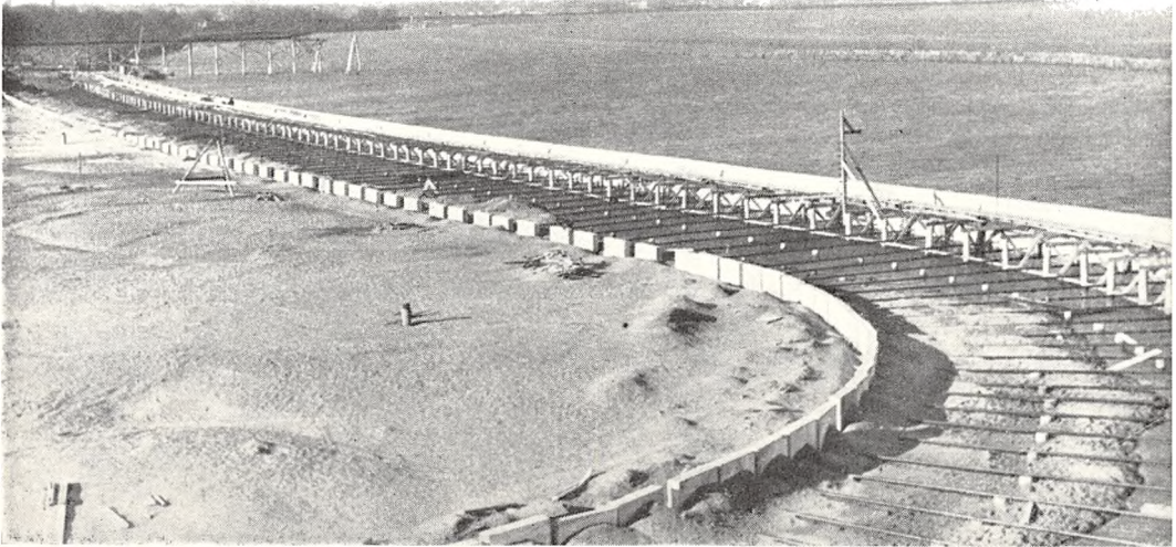
Dansk Ingeniørarbejde i Beograd: Inddæmning og Opfyldning (Kampsax m. fl.)
