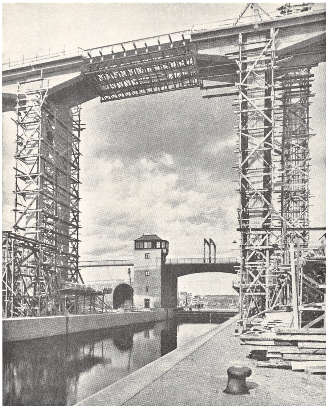
Skanstullbroen i Stockholm, bygget af Monberg & Thorsen
