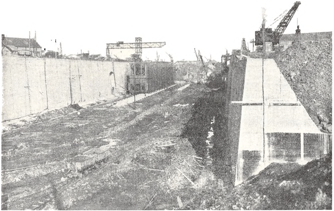
Dok i St. Nazaire. Bygget af Christiani & Nielsen
