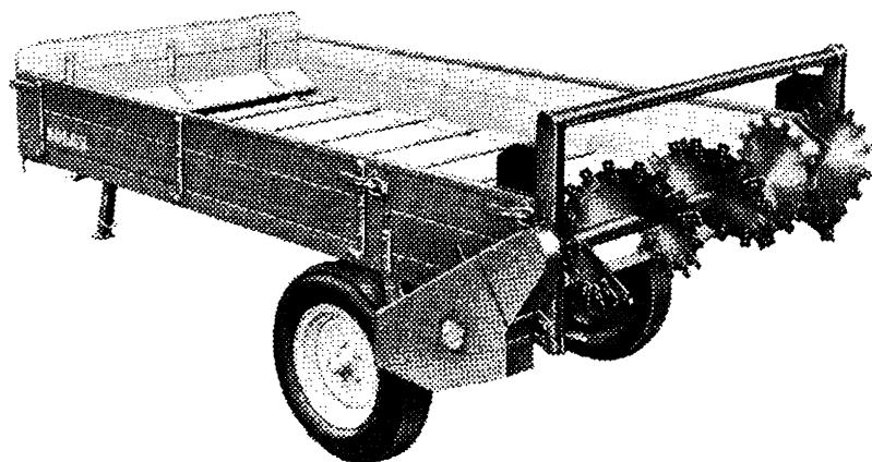
GS-6 Kombi med aftageligt spredeaggregat. Den ideelle kombination af staldgød- ningsspreder og 2-hjulet vogn
