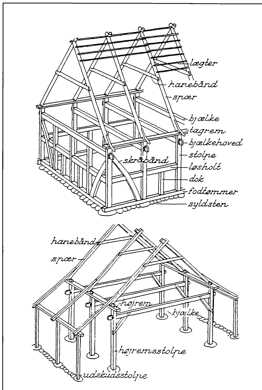
Øverst: Et østjysk eksempel på »almindelig« dansk bindingsværk. Nederst: Den særlige nordvestjyske udgave af bindingsværk – højremkonstruktionen – som huset i Ejerslev er bygget med. Tegningerne er fra Bjarne Stoklunds bog »Bondegård og byggeskik«.
