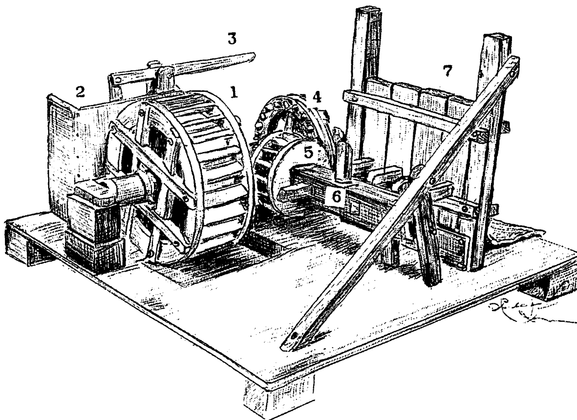
Model af No Stampemølle. Stampemøllen har navn efter stamperne, store egeplanker, som i No vejede 200 kilo pr. stk. De løftedes 30 cm og faldt med stor kraft ned på vadmestøjet. Behandlingen varede to timer. Johan Andersen kaldte dem "mine grå heste". Tegning i Jon Høgh: "No Stampemølle" (1996). 1. Vandhjul - 2. Stigbord - 3. Håndtag til at løfte stigbord - 4. Gravhjul - knaghjul - 5. Stampedrev (stokkedrev) - 6. Stampeaksel - 7. Stamperne.
