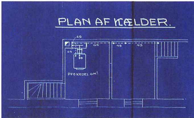
Fig. 2. Plan over kælder med centralvarmeanlæg i Gl. Ankerhus. Centralfyret, hvor bøger af Andersen Nexø gik op i luert, ses øverst t.v. Blåtryk fra 1926 v/ing. Harald Thommesen, København.- Magdalene Lauridsens arkiv, Ankerhus.
