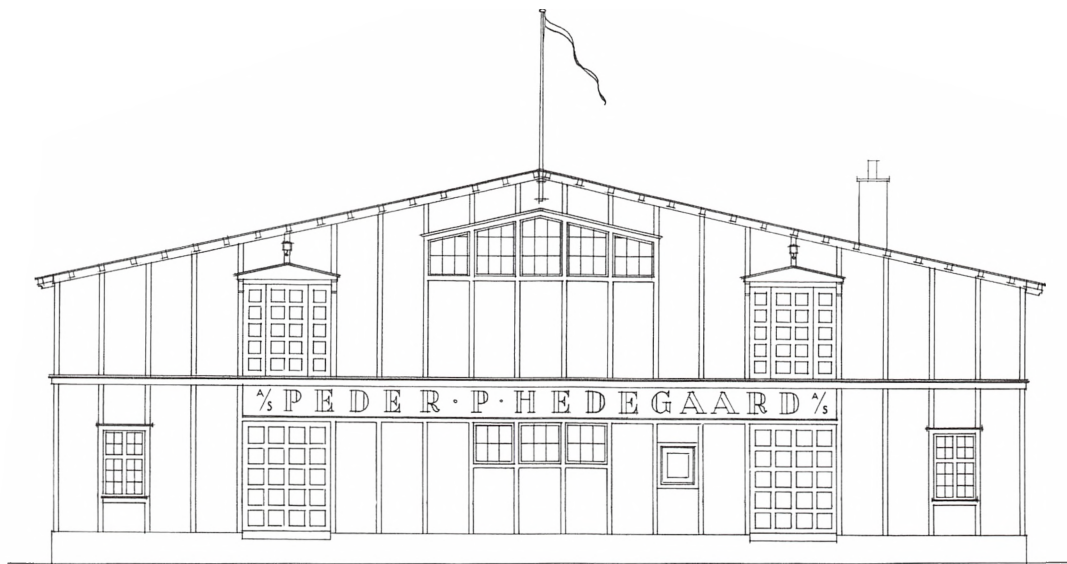
Facade mod Havnen, Syd
