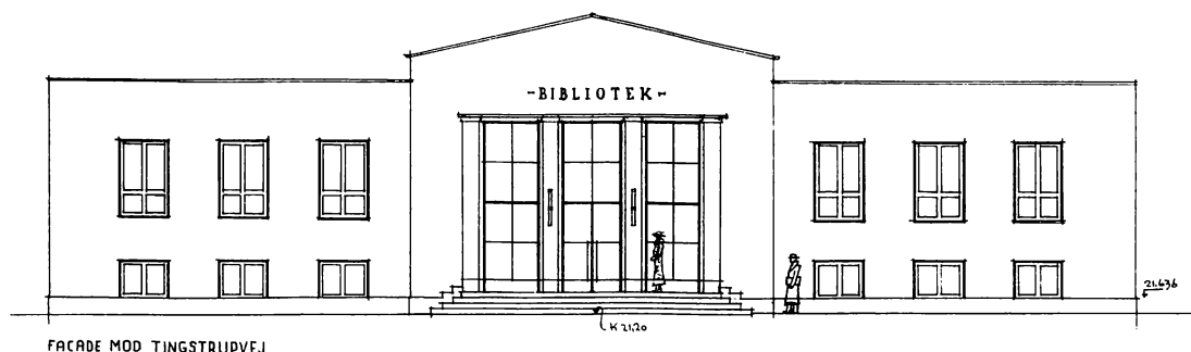
Thisted Bibliotek, 1937.
