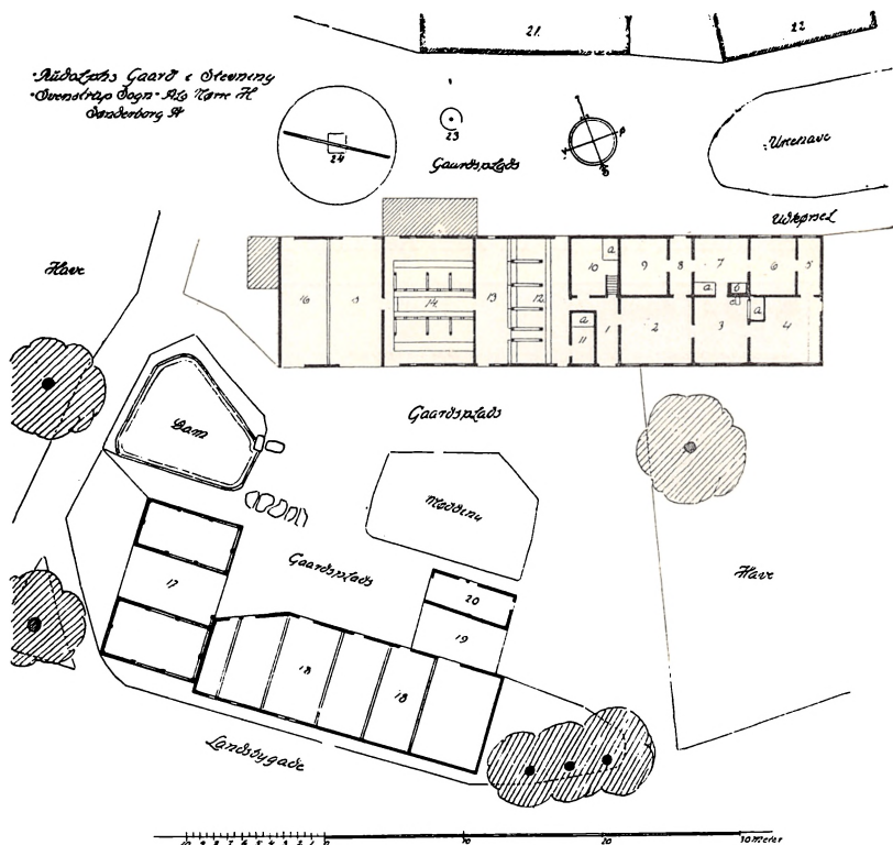
Fig. 12. Grundplan af Rudolphs Gaard i Stevning. (Opmaalt 1923 af Forf.).
