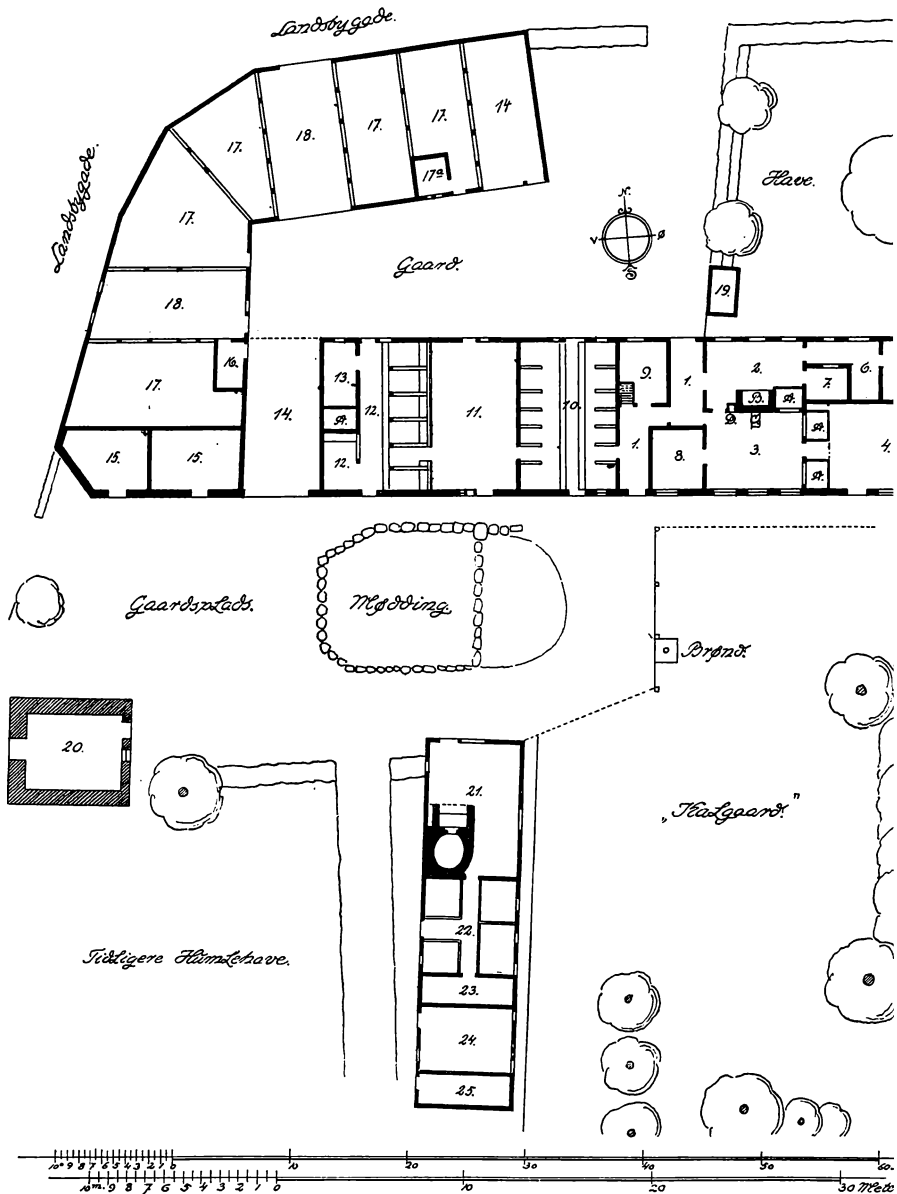
Fig. 13. Grundplan af en Gaard fra Holm. (Maalt af Forf. i 1953).
