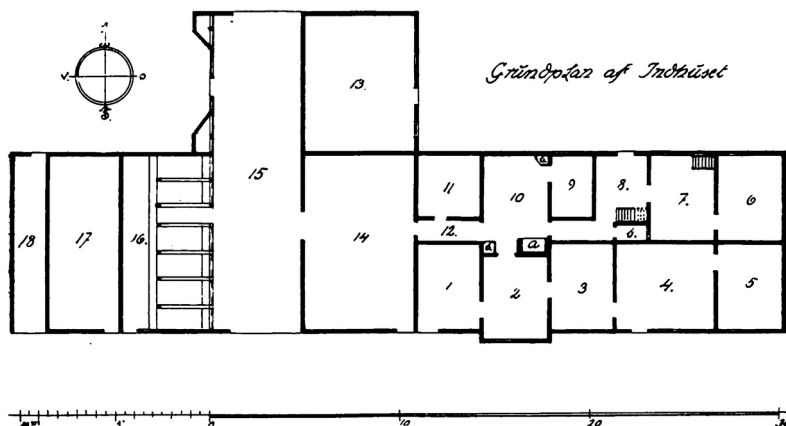
Fig. 6. Grundplan af en Gaard i Fjelby.
