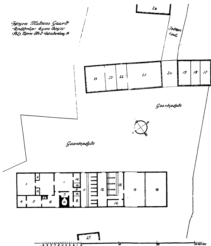
Fig. 9. Grundplan af en Gaard i Sjellerup. (Tegnet efter Matrikelkort og en Skizze, meddelt af Jørgen Nielsen i Guderup). 1) Framgulo. 2) Dørns. 3) Pisel 4) Mælkekammer. 5) Lilledøns. 6) Køkken. 7) Bagehus. 8) Pige-kammer. 9) Gang. 10) Karlekammer. 11) Kostald. 12) Lille Lo. 13) Hestestald. 14) Føllade. 15) Store Lo. 16) Kornkiste. 17) Redskabsrum. 18) Huggetlade. 19) Halmlade. 20) Gennemfart. 21) Kornkiste. 22) Gaasesti. 23) Faare- og Kalbesti. 24) Hølade. 26) Svin og Høns. 27) Trælade (Brændsel). a) Alkover. b) Aaben Skorsten. c) Bagerovn.
