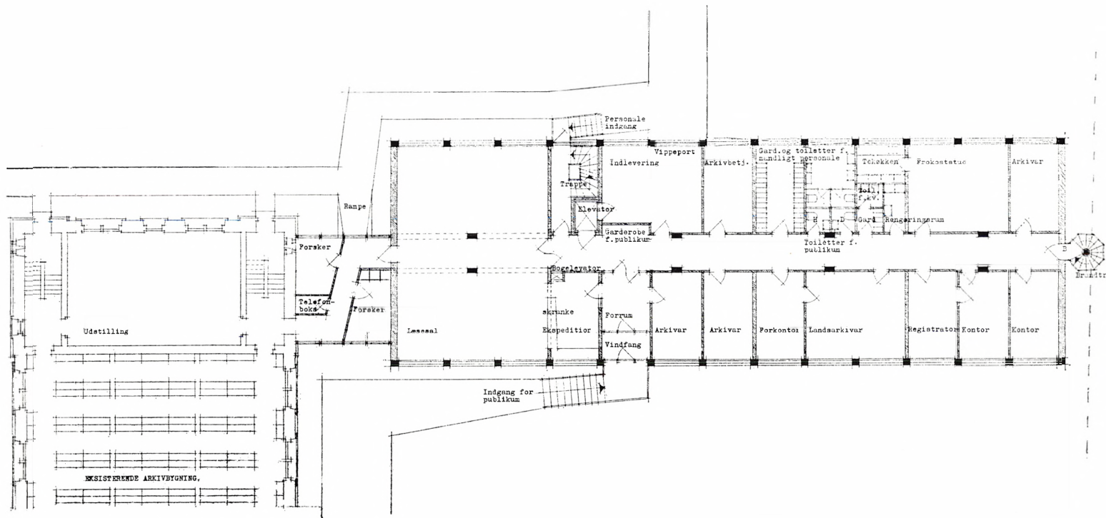
Udkast til kontor- og læsesalsetagen i det nye landsarkiv i Viborg. (Kgl. bygningsinspektør R.Teschl).
