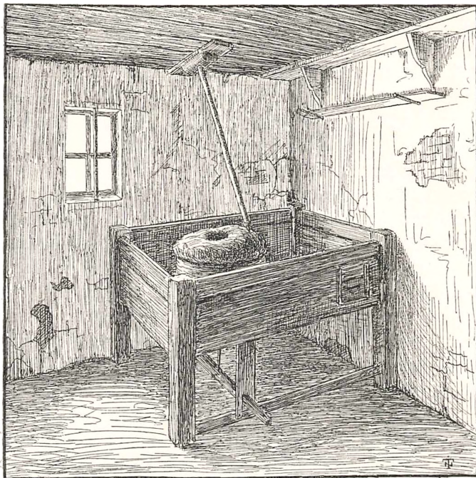
MALTKVÆRN I LILLE RAVNEBJERGHUS Tegning af Niels Jokum Termansen.
