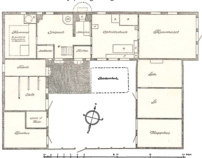
GRUNDPLAN AF LILLE RAVNEBJERGHUS Tegning af M. P. Madsen.
