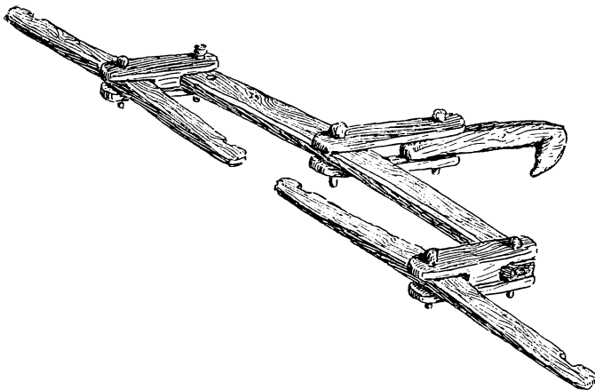
TRÆKTØJ (HAMMELSTØJ) AF TRÆ
