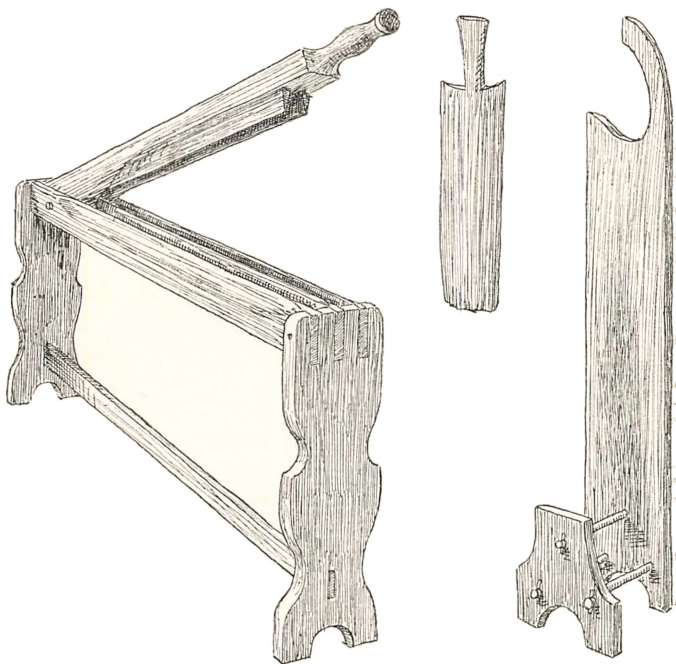
BRYDE, SKÆTTEHAAND OG SKÆTTEFOD
