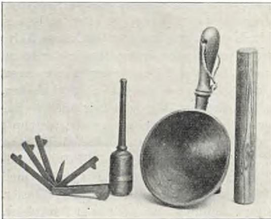
Til venstre: Ladejærn med Kølle. Til højre: Toldkop, hvormed Mølleren toldede af Kornet, og Stok til at stryge over Toldkoppen med.
