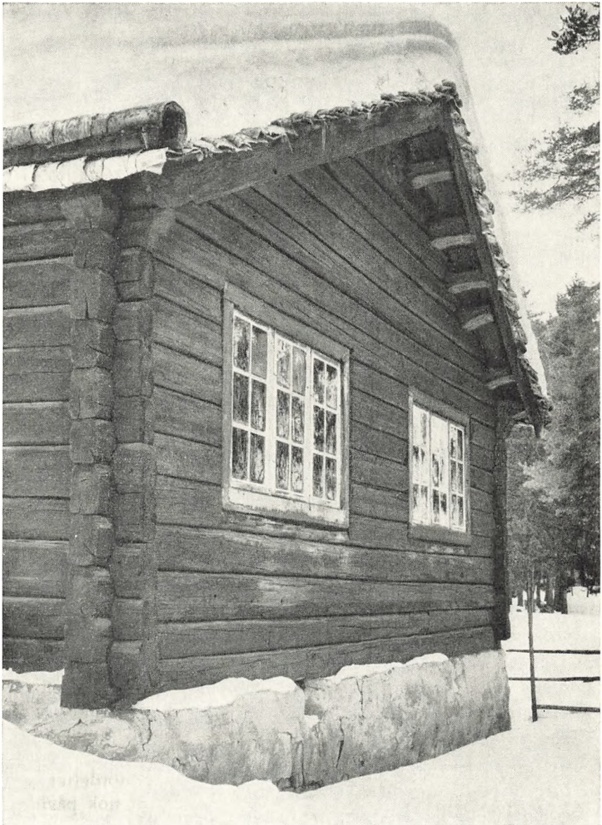
På en sommerstue fra Kilde i Østerdal ses den tagkonstruktion, der betegnes som åstaket. Åsene rider på stokkene i gavlvæggen og når helt frem til tagets kant. (Norsk Folkemuseum fot.).
