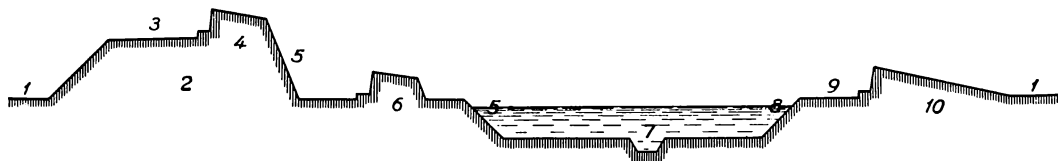
Afb. 11. Skematisk Fremstilling af et bastioneret Anlægs Profil i udviklet Form. 1 Terrainhøjde. 2 Hovedvold. 3. Voldgang. 4. Brjstværn med Banket. 5 Escarpe. 6 Faussebraie. 7 Grav med Cunette. 8 Contrescarpe. 9 Dækket Vej. 10 Glacis. O. E. Christensen del.
