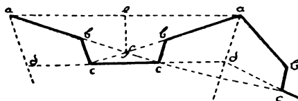
Afb. 10. Skematisk Fremstilling af det bastionerede Anlægs Front i enkei Form. a-a Grundlinie (3-400 m.) a-e \frac{1}{2} Grundlinie (150-200 m). c-f Lodlinie ( \frac{1}{4} - \frac{1}{6} af a-a). a-b Farcer ( \frac{1}{3} af a-a). b-c Flanker. b-c-b 90^\circ . b-a-b Saillant eller Bastionsvinkel, ikke mindre end 60^\circ . c-c Kurtine. abcbca Bastioneret Front. ac Defence- eller Bestrygningslinien. afa Tenaillevinkel. c Kurtinepunkter. cc Bastionshalsen. dd Indre Polygon eller Indre Grundlinie. Jvf. Afb. 93. Efter E. Langenskiöld.
