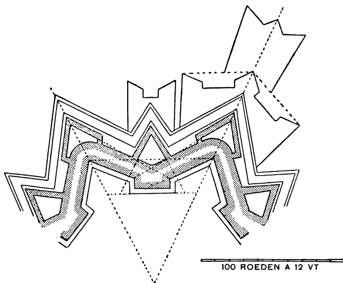
Afb. 12. Det ældre nederlandske System i dets modne Form paa Grundlag af de af S. Marolois og A. Freitag udarbejdede Forbedringer, bl. a. med Horn- og Kronværker. Efter W. H. Schukking.
