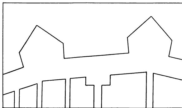
Afb. 28. Plads mod Fæstningsterrainet i Frederikssodde 1657 O. E. Christensen del.
