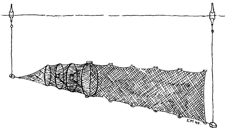
En Kasteruse (til Torsk). Tegning af E. Mikkelsen.
