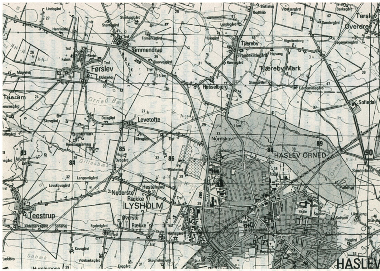
Udsnit af Geodætisk instituts 2 cm-kort. © Kort og Matrikelstyrelsen (A. 140-99).
