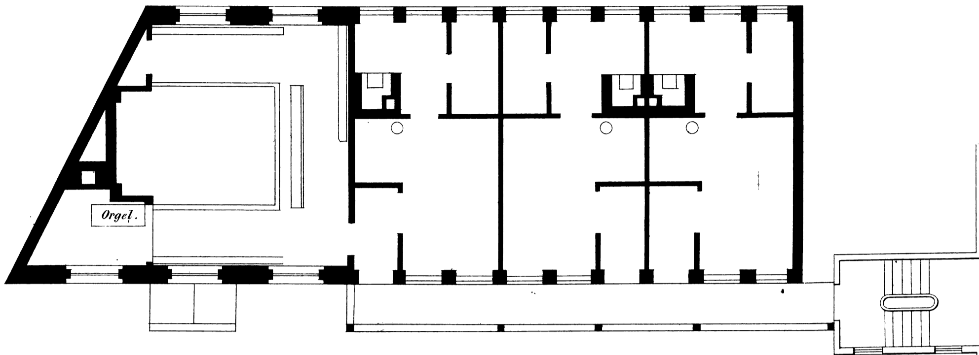
Plan af 1ste Sal.
